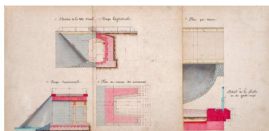
Bief de Chantes - Construction d'une dérivation éclusée, d'un barrage mobile et d'un chemin de halage. Ponceau sur le ruisseau de la Fontaine (1878) : Plans, coupes, élévations et détails. Phot. Jérôme Mongreville, Autr. Gustave Bouvaist IVR43_20207000093NUC4A
