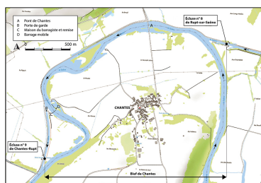
Plan de localisation (1/50 000). Extrait du ScanExpress standard © IGN 2018 Dess. Bertrand Turina IVR43_20207000774NUDA
