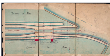
Bief de Chantes - Plan des abords de l'écluse à sas (1878). Phot. Jérôme Mongreville, Autr. Gustave Bouvaist IVR43_20207000092NUC4A
