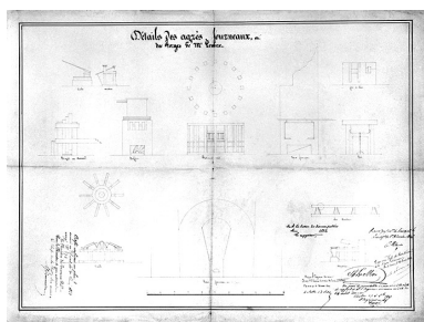
Détail des agrès, fourneaux, etc. des forges de Mr Lemire. Phot. Jérôme Mongreville IVR43_19963900207X
