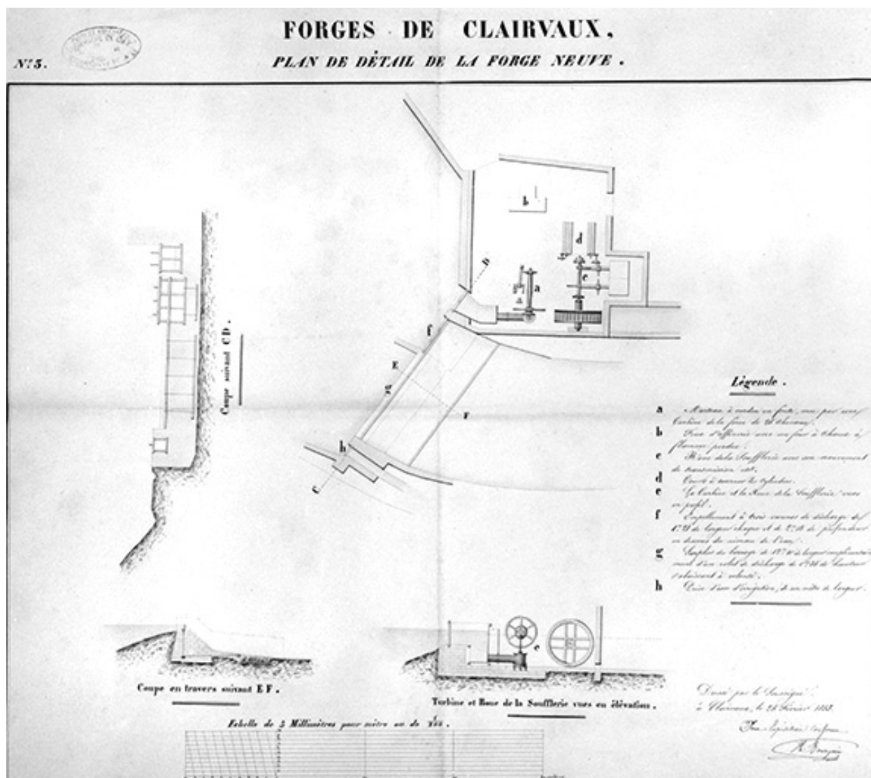
Plan de détail de la forge neuve.
