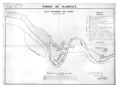
Plan d'ensemble des usines. Phot. Jérôme Mongreville, Autr. H. Bourquin IVR43_19963900210X
