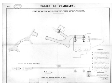
Plan de détail de l'ancienne forge et du cylindre. Phot. Jérôme Mongreville, Autr. H. Bourquin IVR43_19963900208X
