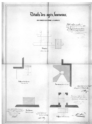
Détail des agrès, fourneaux, des forges de Mr Lemire à Clairvaux. Phot. Jérôme Mongreville IVR43_19963900206X
