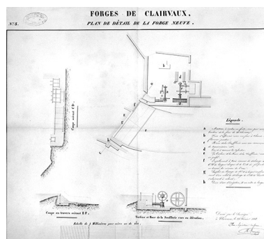
Plan de détail de la forge neuve. Phot. Jérôme Mongreville, Autr. H. Bourquin IVR43_19963900209X
