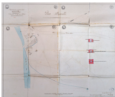
Ringuelet. Plan d'ensemble [de la conduite de la source Javelot]. 1841. Autr. Charles Alexandre Ringuelet, Repro. Jérôme Mongreville IVR43_20197000032NUC4A
