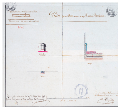
Ringuelet. Plan pour l'établissement de sept bornes fontaines. 1841. Autr. Charles Alexandre Ringuelet, Repro. Jérôme Mongreville IVR43_20197000029NUC4A
