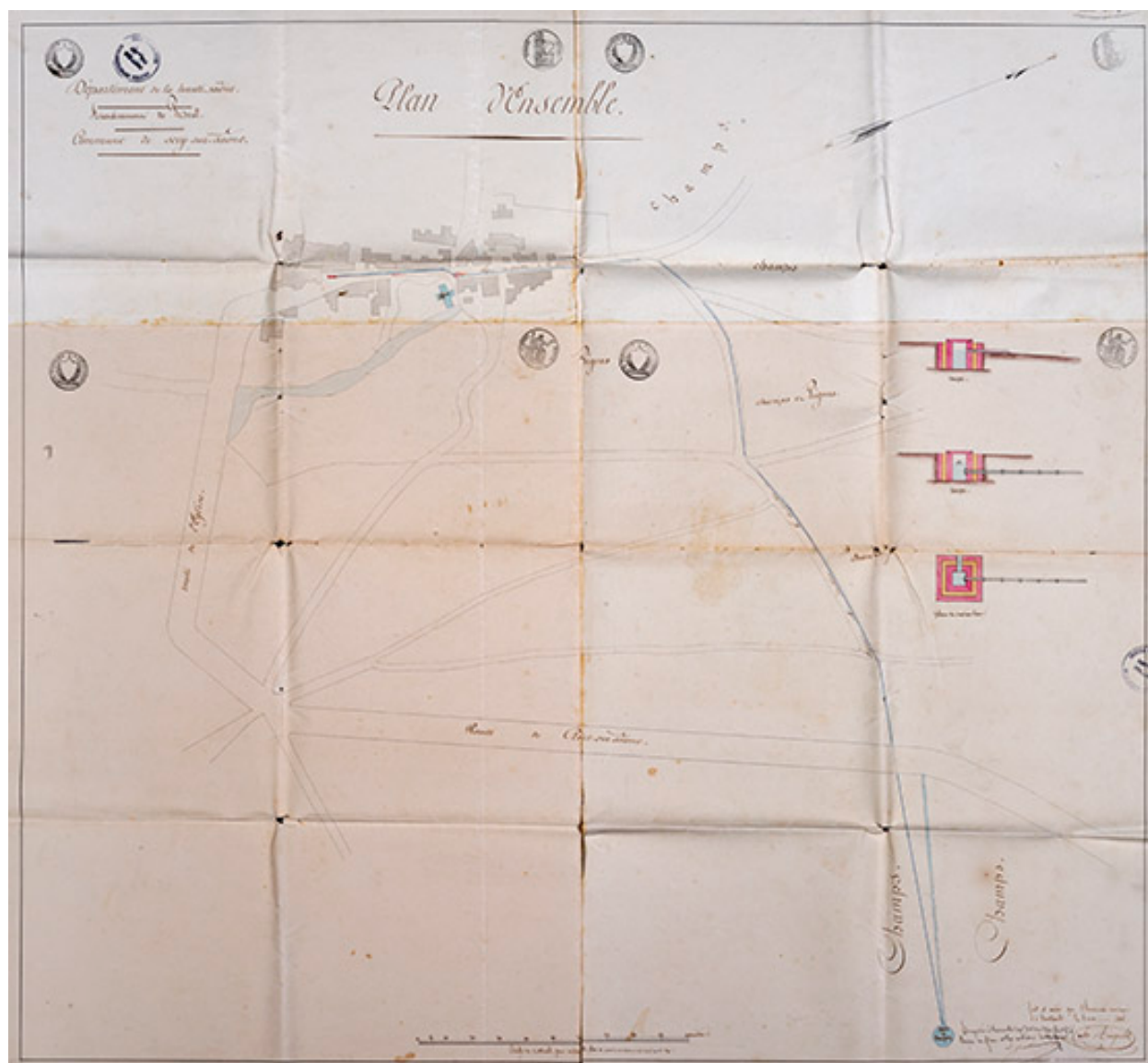
Ringuelet. Plan d'ensemble [de la conduite de la source Beaufroy]. 1841.
