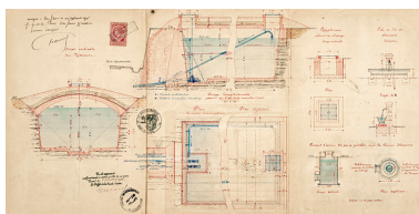
[Plan, coupe et élévation du réservoir de La Prouse]. 1906. Phot. Jérôme Mongreville IVR43_20197000010NUC4A
