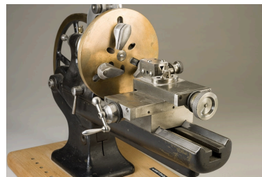
Perche, chariot porte-outil et porte-pièce, vu de trois quarts. Phot. Marc Loukachine IVR43_20122500077NUC4A
