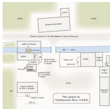
Plan général de l'usine d'horlogerie Roux, dessin. D'après un calque de 1858, échelle 1/100, conservé aux AD Doubs (432 S 6). Dess. Mathias Papigny IVR43_20142500604NUDA
