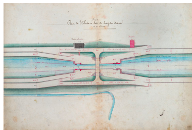
Achèvement de la dérivation de Scey-sur-Saône, écluse à sas - Plans, élévations, coupes et détails (1876). Phot. Jérôme Mongreville, Autr. Gustave Bouvaist IVR43_20207000079NUC4A
