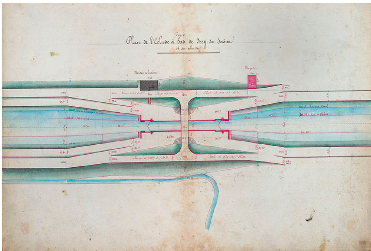
Achèvement de la dérivation de Scey-sur-Saône, écluse à sas - Plans, élévations, coupes et détails (1876).
