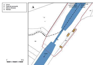
Plan-masse et de situation. Extrait du plan cadastral, 2019. Dess. Bertrand Turina IVR43_20197000194NUDA
