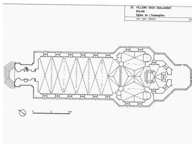
Plan au sol. Phot. Dominique et Sancey Dominguez IVR43_19792500012V
