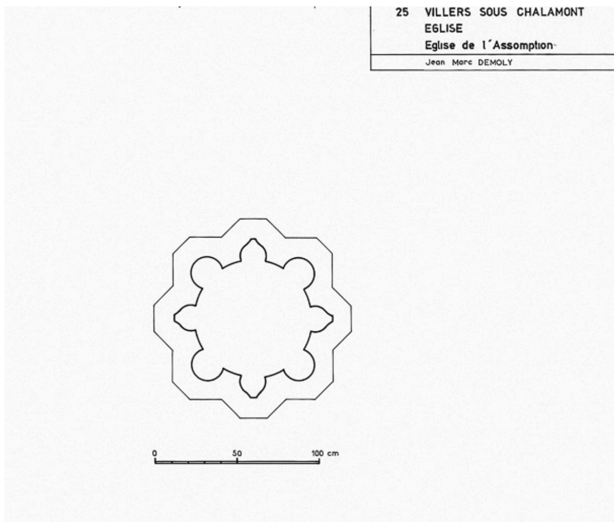
Détail : coupe d'un pilier de la croisée du transept.
