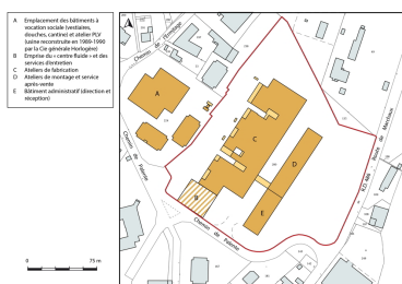
Plan-masse et de situation. Extrait du plan cadastral, 2019. Dess. Bertrand Turina IVR43_20192501114NUDA
