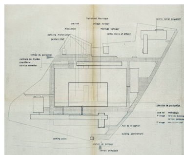
Plan-masse de l'usine, 1957. IVR43_20192500050NUC4A
