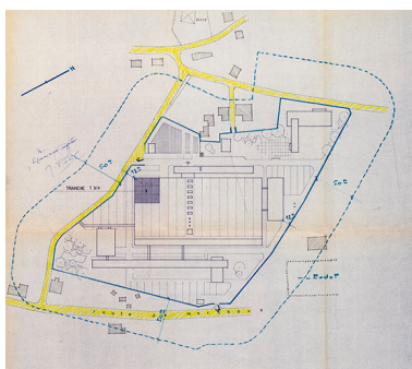
Usine de Palente. Plan-masse, 1957. IVR43_20192500049NUC4A
