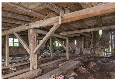
Entrepôt industriel. Rez-de-chaussée. Phot. Jérôme Mongreville IVR43_20142501291NUC4A
