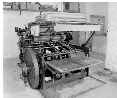
Partie arrière de la machine. A la sortie du cylindre, le receveur mécanique à raquettes dépose la feuille sur la table de réception. Phot. Jérôme Mongreville IVR43_20023900365X
