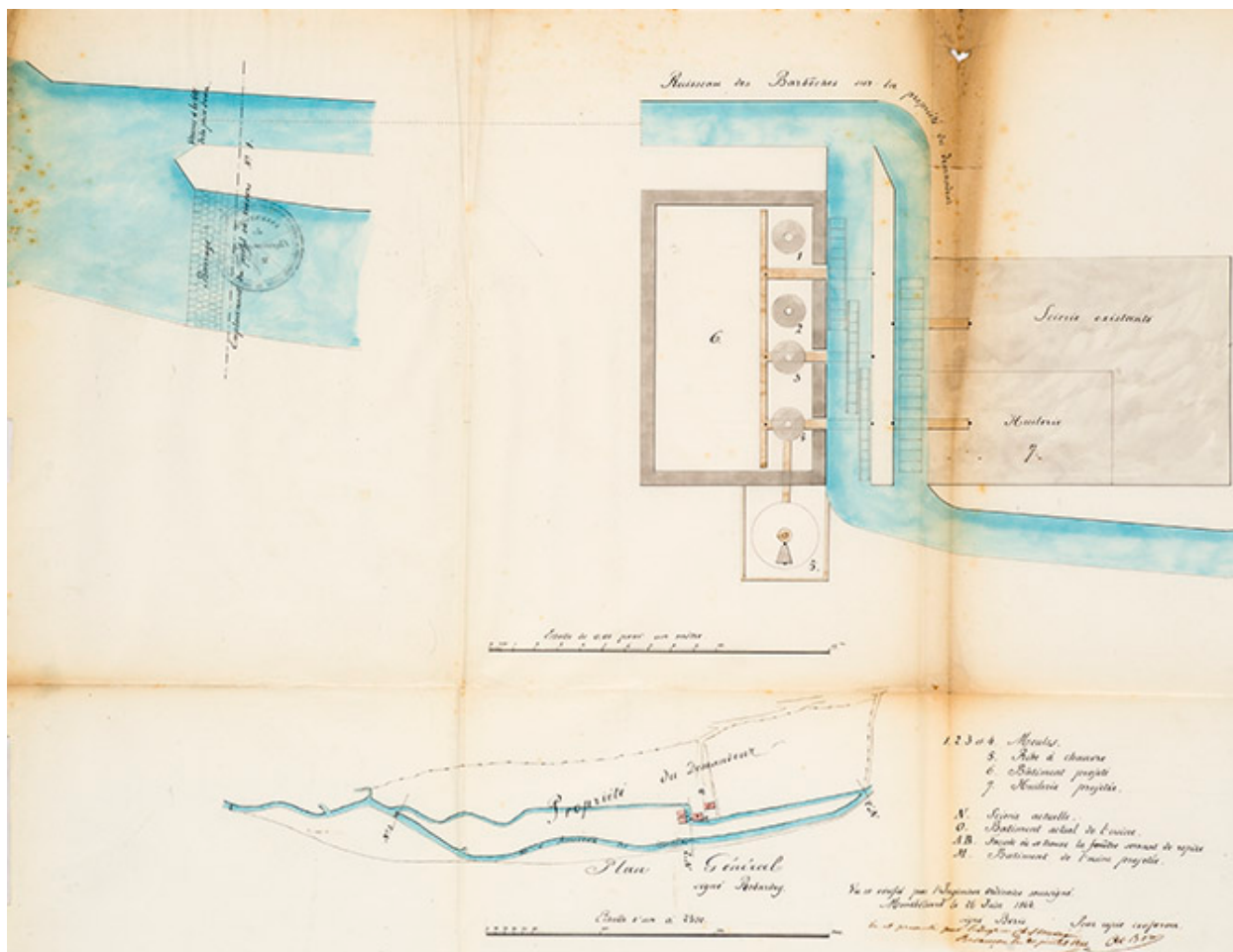
Plan général [plan-masse et de situation], 1844.
