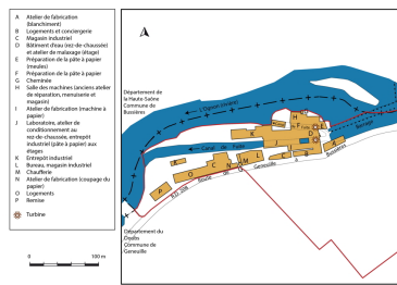
Plan-masse. Extrait du plan cadastral, 2019. Dess. Bertrand Turina IVR43_20192501038NUDA
