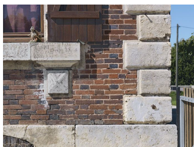
Maison éclusière : chaîne d'angle et encadrement de la fenêtre. Phot. Thierry Kuntz IVR26_20118900175NUC4A
