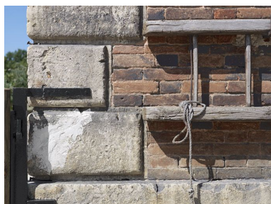
Maison éclusière : détail de la chaîne d'angle et de l'échelle fixée sur le côté. Phot. Thierry Kuntz IVR26_20118900171NUC4A
