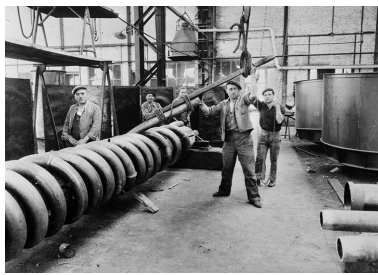
Atelier de réparation : réfection et mise en place de la tuyauterie d'un appareil sécheur de la soudière. Phot. Jérôme Mongreville, Phot. Charnotet IVR43_19903900069X
