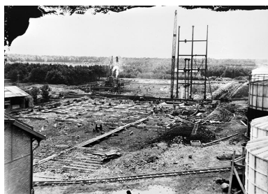
Construction de l'atelier de caustification : pose de la 1ère travée de l'ossature métallique, en 1930. Phot. Jérôme Mongreville, Autr. photographe) NEPASUTILISERCharnotet (? IVR43_19903900044X
