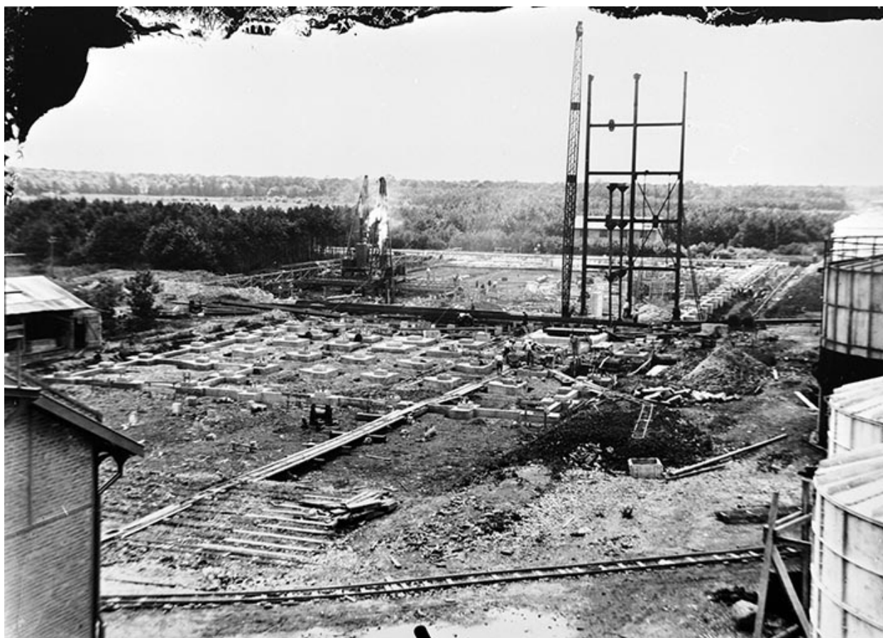
Construction de l'atelier de caustification : pose de la 1ère travée de l'ossature métallique, en 1930.
