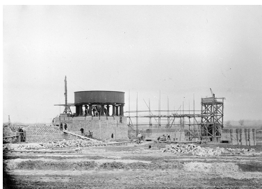
Construction des fours à chaux : base du 1er four.
