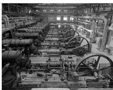
Soudière (10), salle des machines : vue d'ensemble des pompes à gaz. Phot. Yves Sancey IVR43_19893900415X
