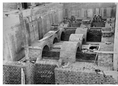
Atelier du chlorure de calcium : construction des pots. Phot. Jérôme Mongreville, Phot. Charnotet IVR43_19903900064X
