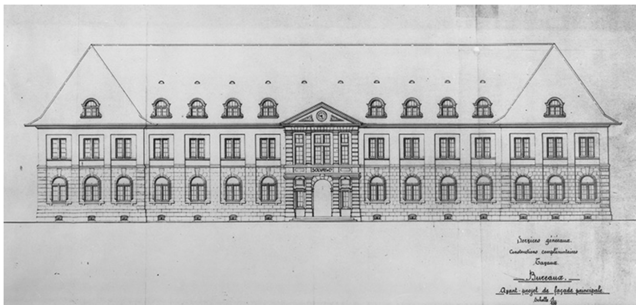
Bureaux. Avant-projet de la façade principale. B.17 001.
