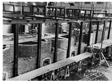
Atelier de caustification : construction des pots (batterie n° 2). Phot. Jérôme Mongreville, Phot. Charnotet IVR43_19903900061X
