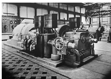
Bâtiment des générateurs : turboalternateur Rateau - Brown Boveri.
