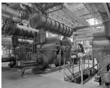
Soudière, salle des machines : arrière de la pompe n° 4. De gauche à droite : axe des compresseurs, compresseurs surmontés d'un séparateur d'humidité (réservoir cylindrique) puis cylindre à vapeur et bielle. Phot. Yves Sancey IVR43_19893900419X
