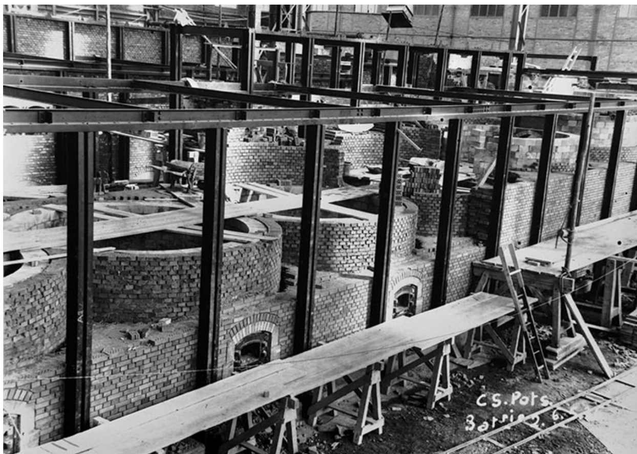
Atelier de caustification : construction des pots (batterie n° 2).
