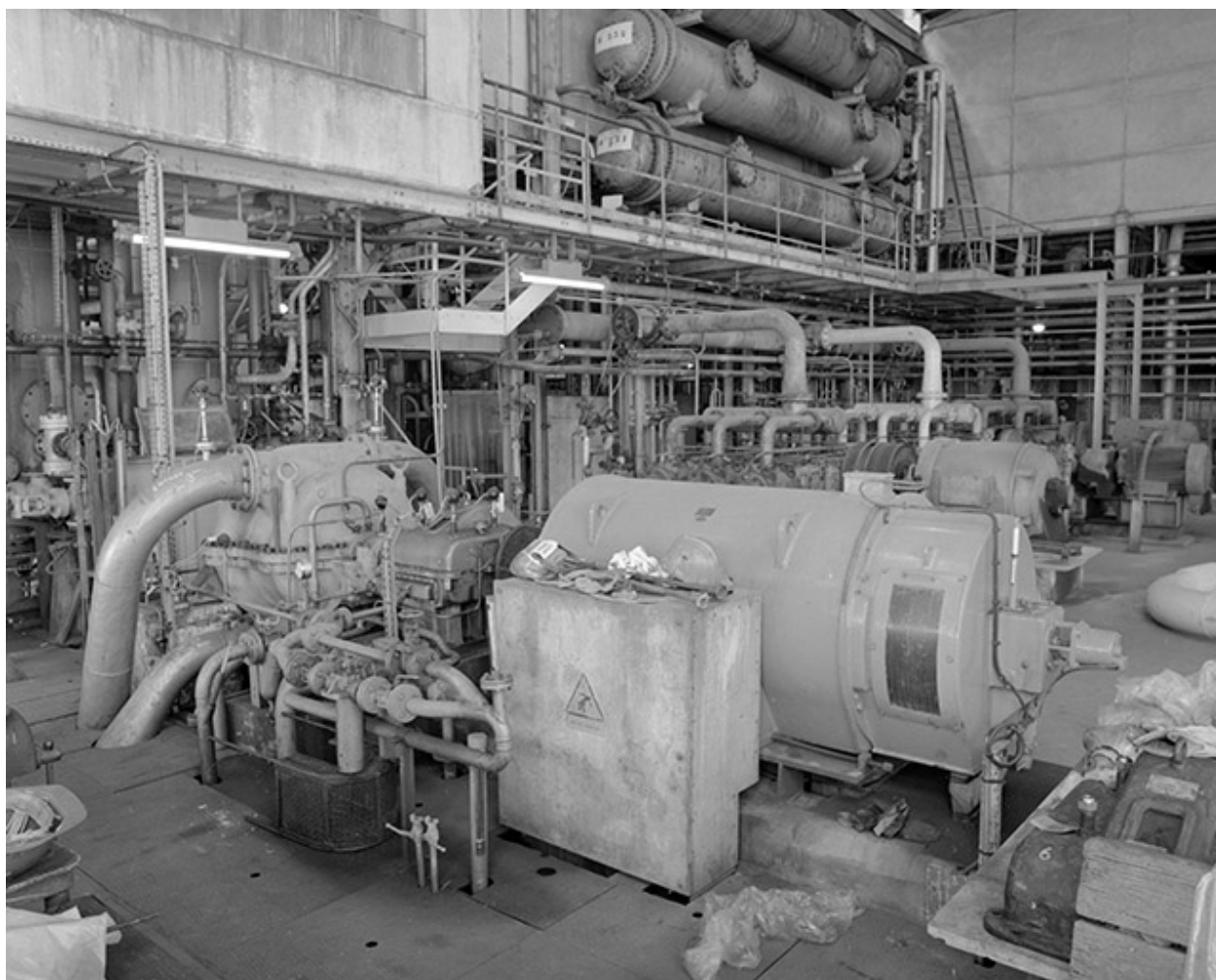
Usine d'électrolyse (37), Salle 3 : soufflante à chlore. De gauche à droite : compresseur (soufflante), variateur de vitesse et moteur électrique.
