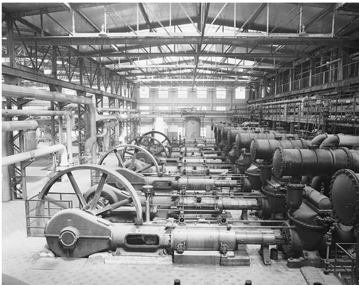
Soudière, salle des machines : vue d'ensemble des pompes à gaz depuis le sud.
