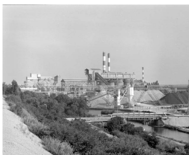
Caisses à soude (13) et fours à chaux (9) vus du haut des bassins de décantation. Phot. Yves Sancey IVR43_19893900381X
