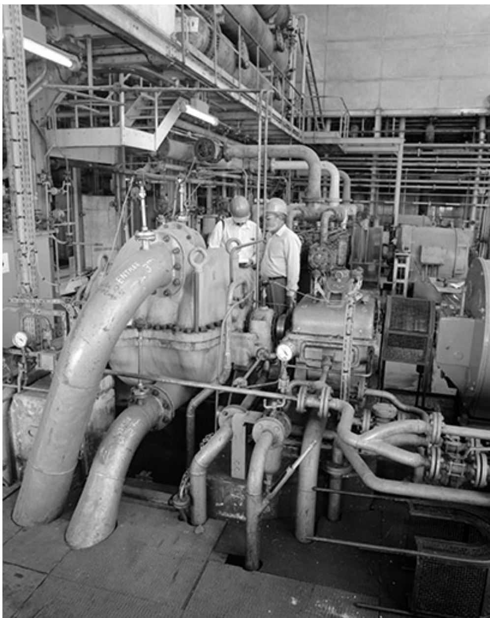
Usine d'électrolyse, Salle 3 : détail du compresseur Rateau et du variateur SACM (vue en hauteur).
