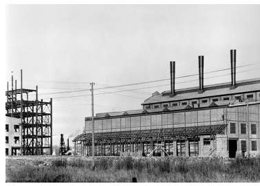
Générateurs de vapeur et d'électricité en construction.
