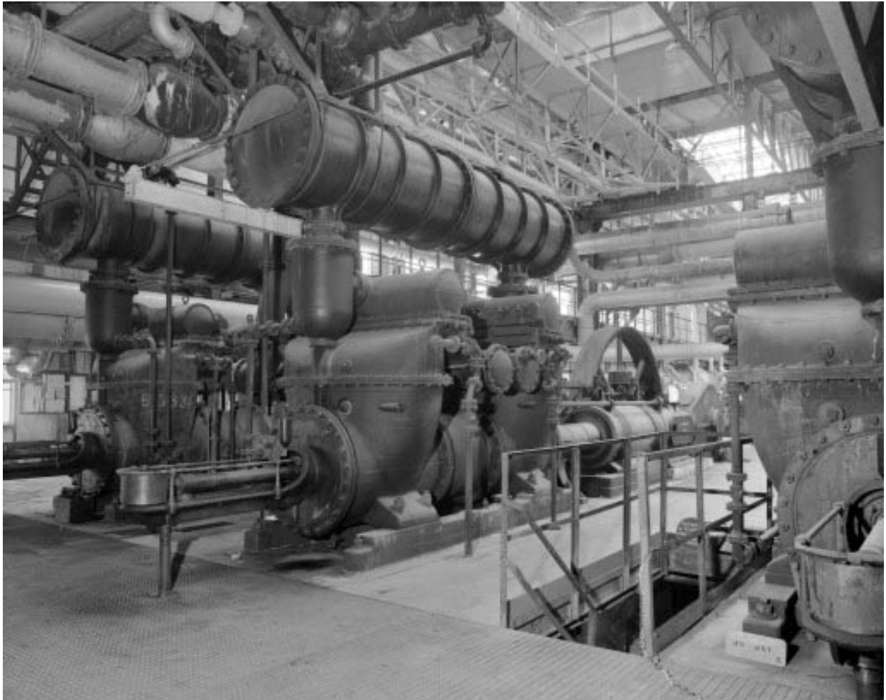
Soudière, salle des machines : arrière de la pompe n° 4. De gauche à droite : axe des compresseurs, compresseurs surmontés d'un séparateur d'humidité (réservoir cylindrique) puis cylindre à vapeur et bielle.
