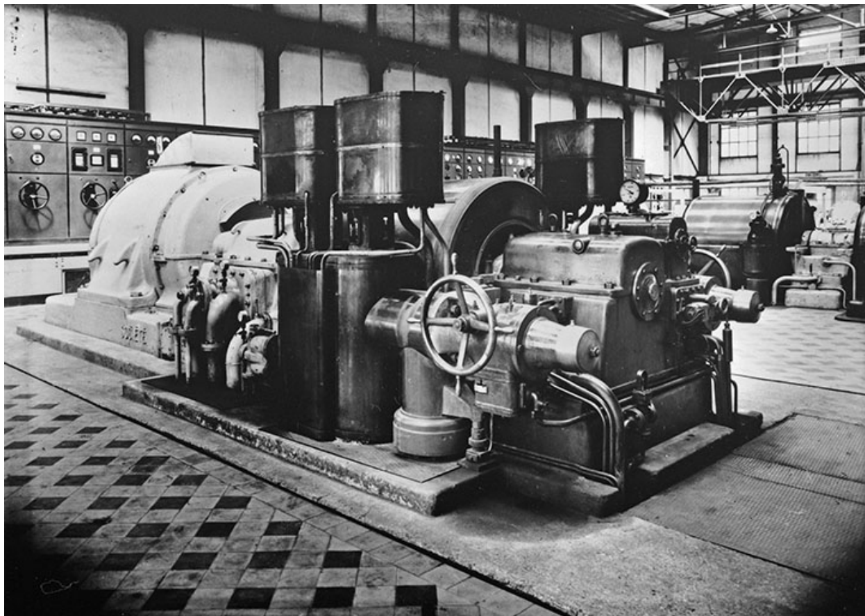
Bâtiment des générateurs : turboalternateur Rateau - Brown Boveri.
