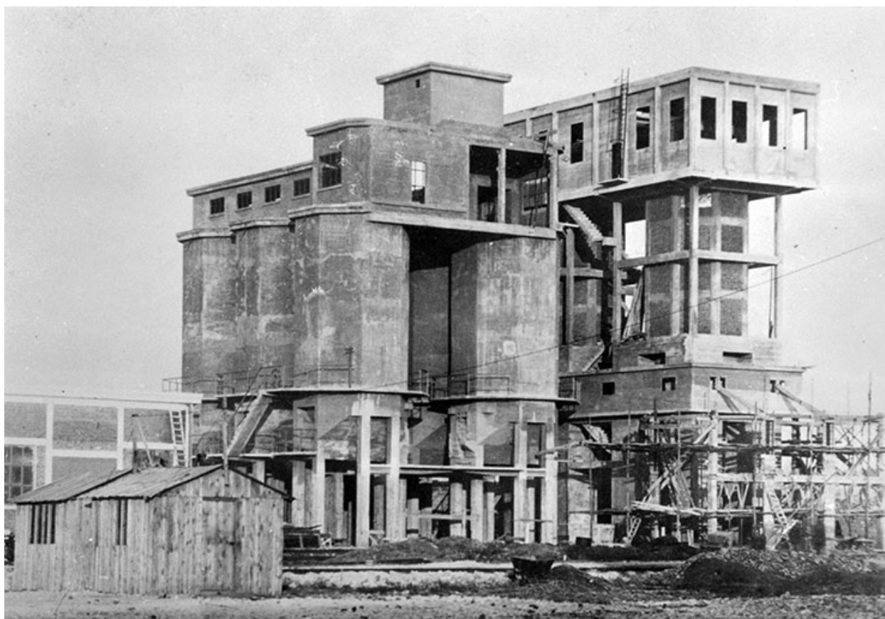
Fours Backmann en construction.
