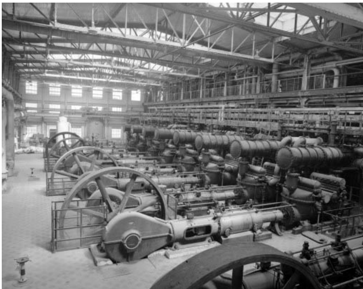
Soudière, salle des machines : vue d'ensemble des pompes à gaz (vue de trois quarts).
