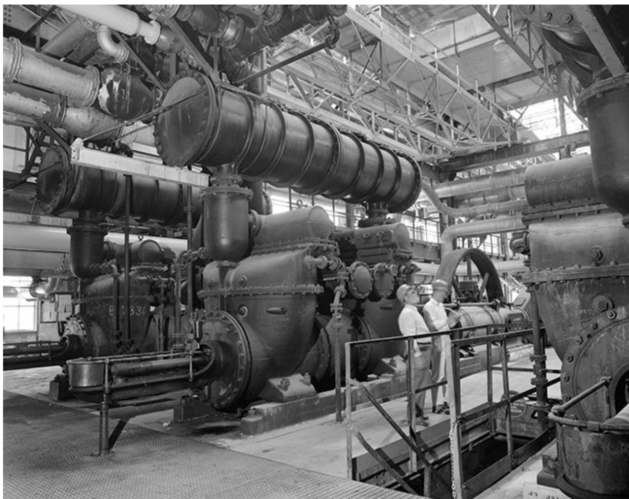
Soudière, salle des machines : arrière de la pompe n° 4 et personnages.
