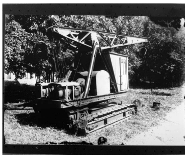
Grue à chenilles. Phot. Jérôme Mongreville, Phot. Charnotet IVR43_19903900078X
