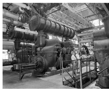
Soudière, salle des machines : arrière de la pompe n° 4 et personnages.
