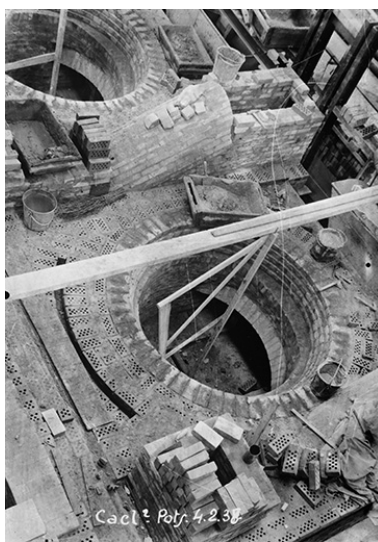
Atelier du chlorure de calcium : construction des pots. Phot. Jérôme Mongreville, Phot. Charnotet IVR43_19903900066X
