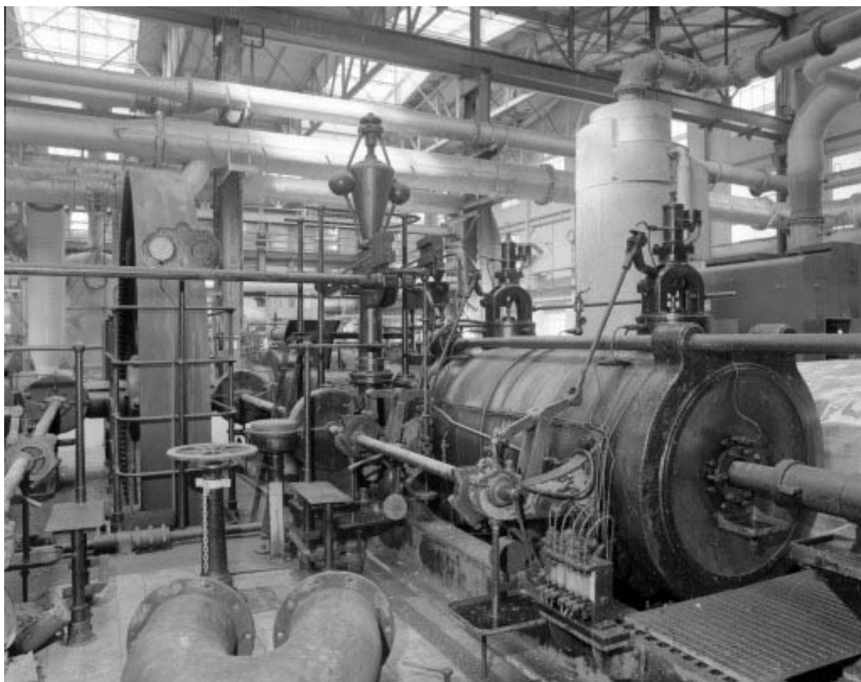
Soudière, salle des machines : volant d'inertie, régulateur à boules et cylindre à vapeur de la pompe n° 1.
