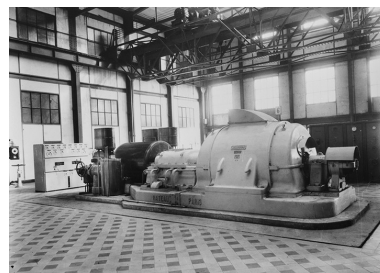
Bâtiment des générateurs : turboalternateur Rateau - Brown Boveri, vers 1940. Phot. Jérôme Mongreville, Phot. Charnotet IVR43_19903900073X
