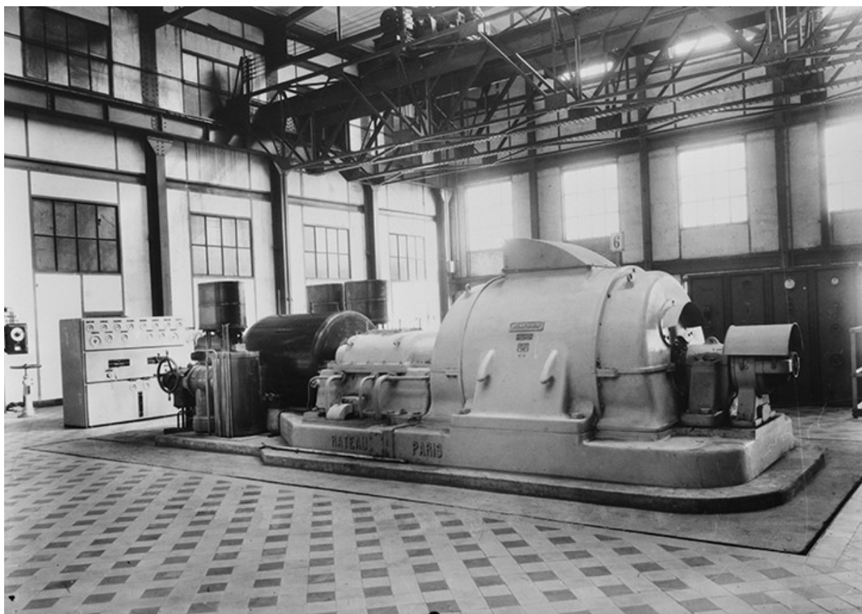
Bâtiment des générateurs : turboalternateur Rateau - Brown Boveri, vers 1940.
