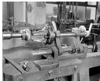
Détail de la fraise et du support de pièce, dans l'atelier d'ébauchage en 1992. Phot. Jérôme Mongreville IVR43_19923900536X
