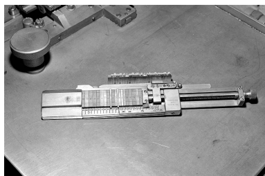
Face supérieure du composteur permettant le centrage des caractères sur la ligne. Le caractère apparaît au recto de chaque matrice ; la ligne-bloc fondue est placée à côté du composteur.
