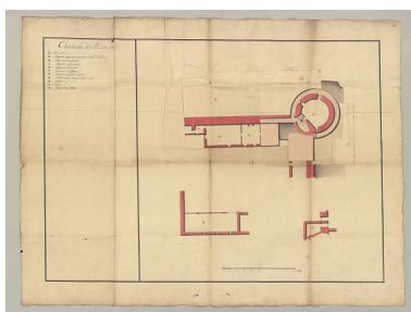
Fol. 18 Château de Blamont : plans (magasin pour 10,000 milliers de poudre) [vue 1]. Autr. auteur inconnu IVR43_20242500024NUC4A
