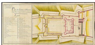
Plan du château de Blamont [sic]. 1747. Autr. Louis de Cormontaigne IVR43_2025250005NUC4A
