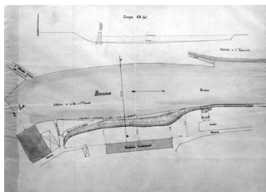
Construction d'un mur [...] Plan et coupe transversale. Phot. Jérôme Mongreville, Autr. Bonnefoy IVR43_19943900432X
