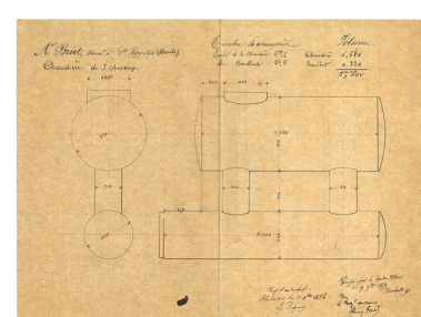
Mr Briot, tann[eu]r à St Hippolyte (Doubs). Chaudière de 3 chevaux, [1859]. Phot. Sonia Dourlot IVR43_20192500895NUC2A
