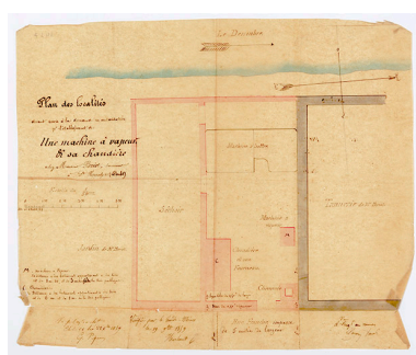
Plan des localités devant servir à la demande en autorisation p[ou]r l'établissement de : une machine à vapeur et sa chaudière chez Monsieur Briot, tannier à St Hippolyte (Doubs), [1859]. Phot. Sonia Dourlot IVR43_20192500857NUC4A
