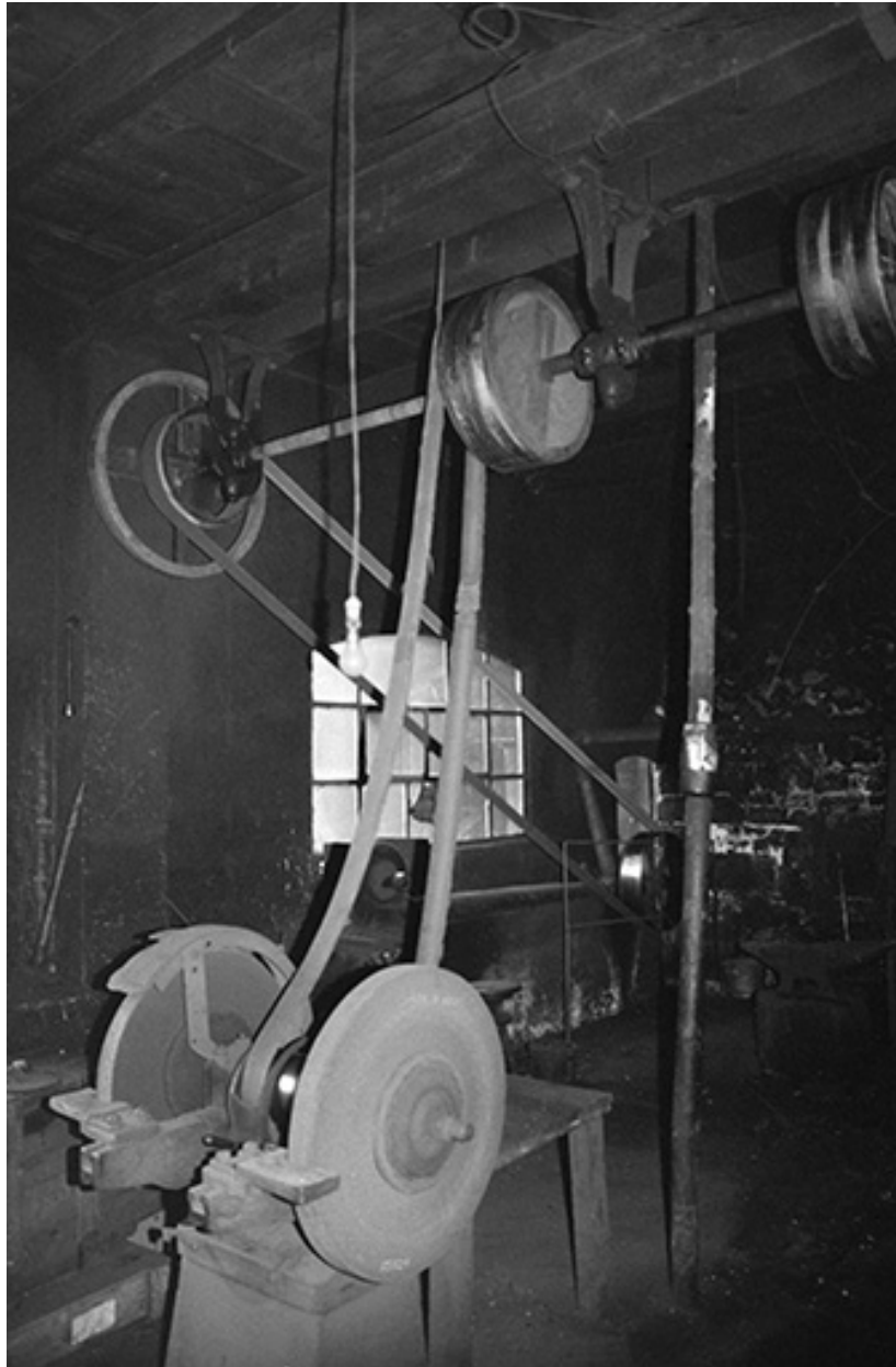
Meules et leur système d'entraînement en 1980.
