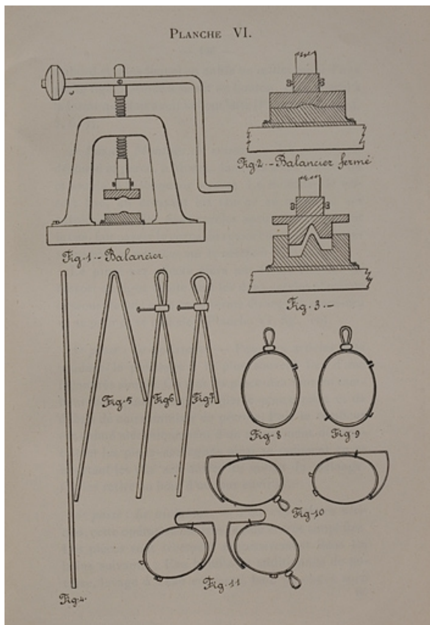
La fabrication des montures [sans soudure], 1913. Dessin imprimé
