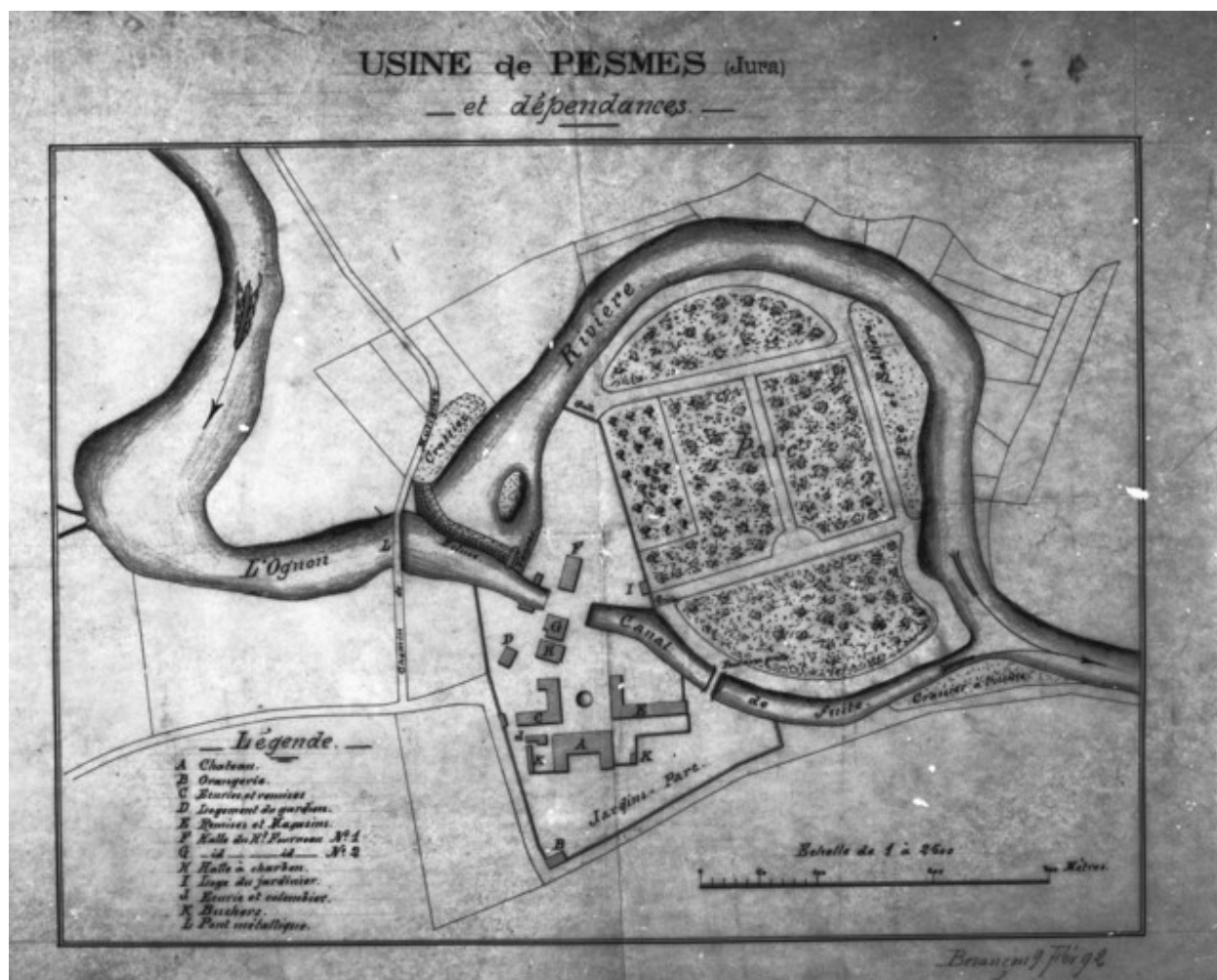
Usine de Pesmes (Jura) et dépendances [plan-masse].
