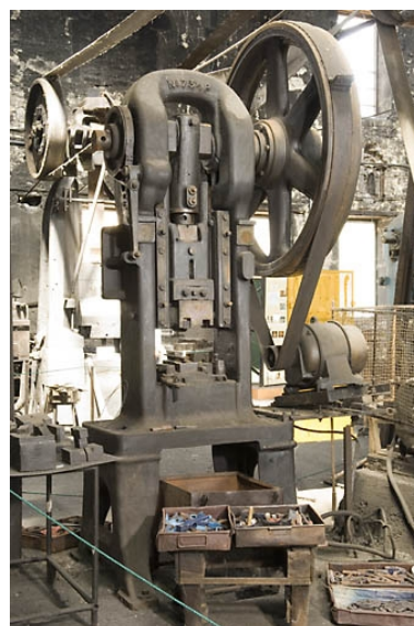
Atelier est. Presse à arcade Bliss. Phot. Jérôme Mongreville IVR43_20087000840NUC2A
