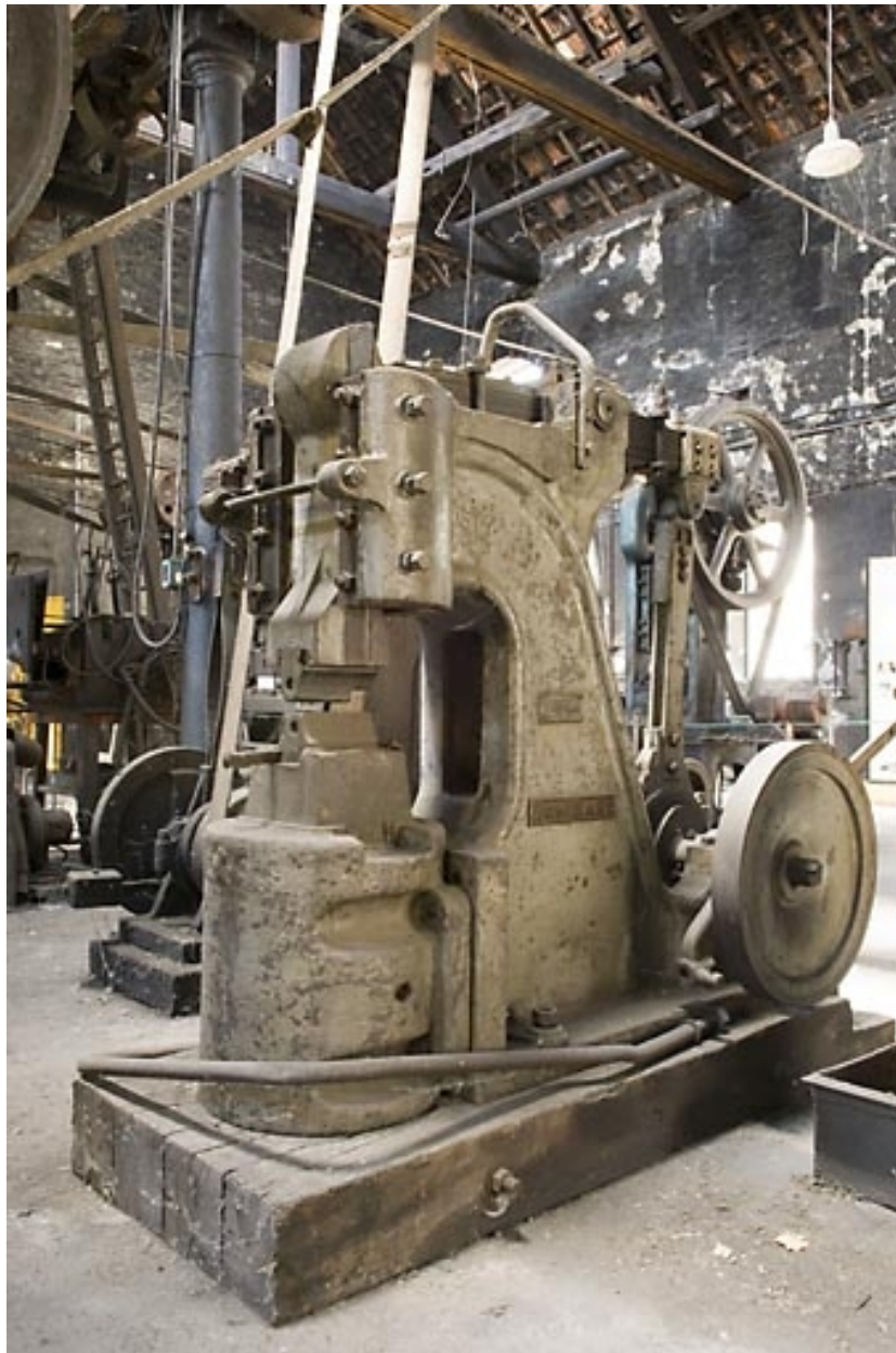
Atelier est. Martinet à ressorts de la Société de Constructions de Montbard.
