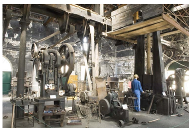
Intérieur de l'atelier est. Vue depuis le sud. Phot. Jérôme Mongreville IVR43_20087000844NUC2A
