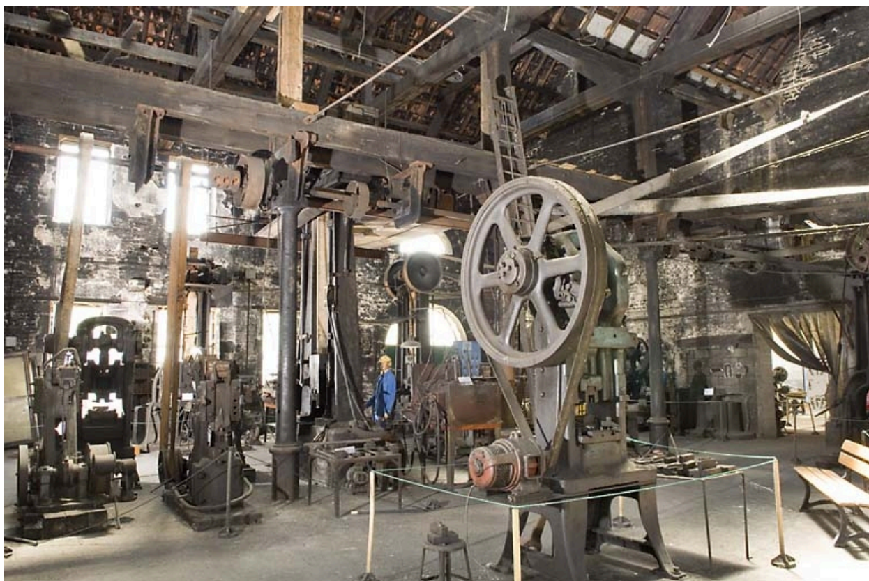
Intérieur de l'atelier est. Vue depuis le nord.
