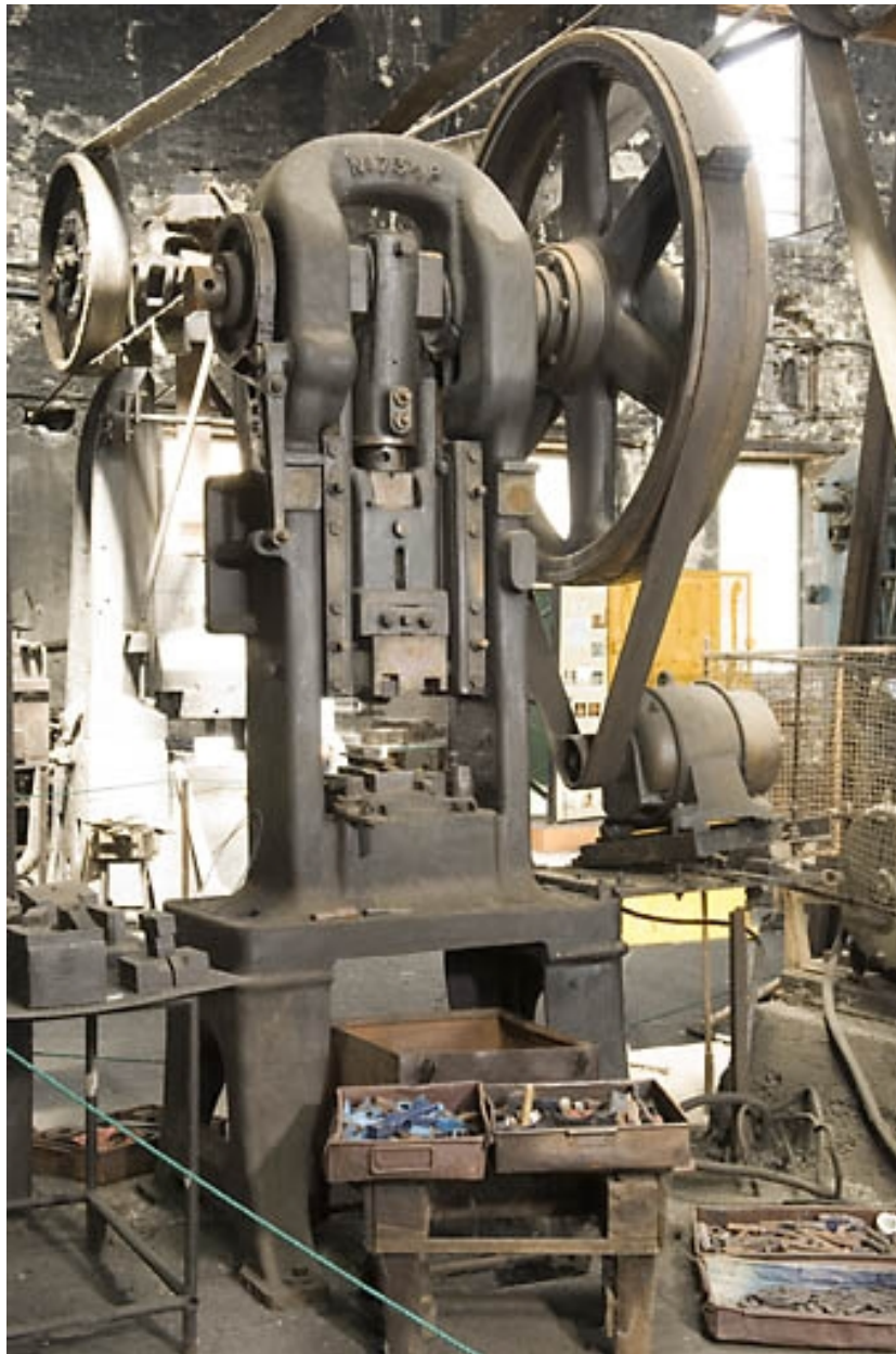
Atelier est. Presse à arcade Bliss.
