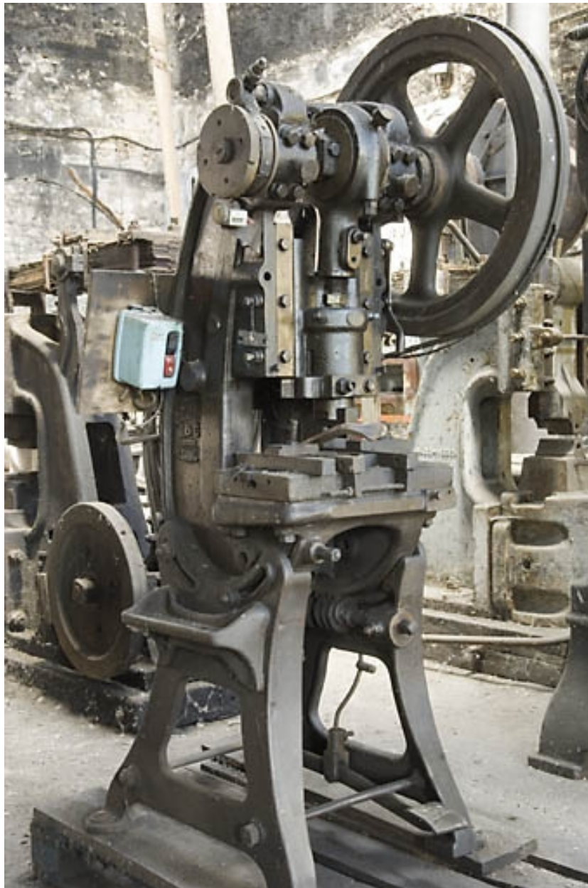
Atelier est. Presse "col de cygne".
