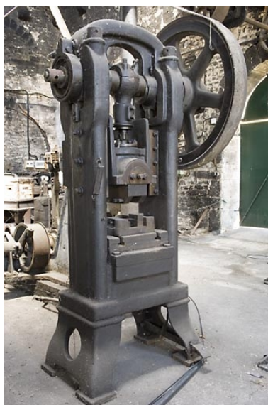
Atelier est. Presse à arcade Perla (Besançon). Phot. Jérôme Mongreville IVR43_20087000833NUC2A
