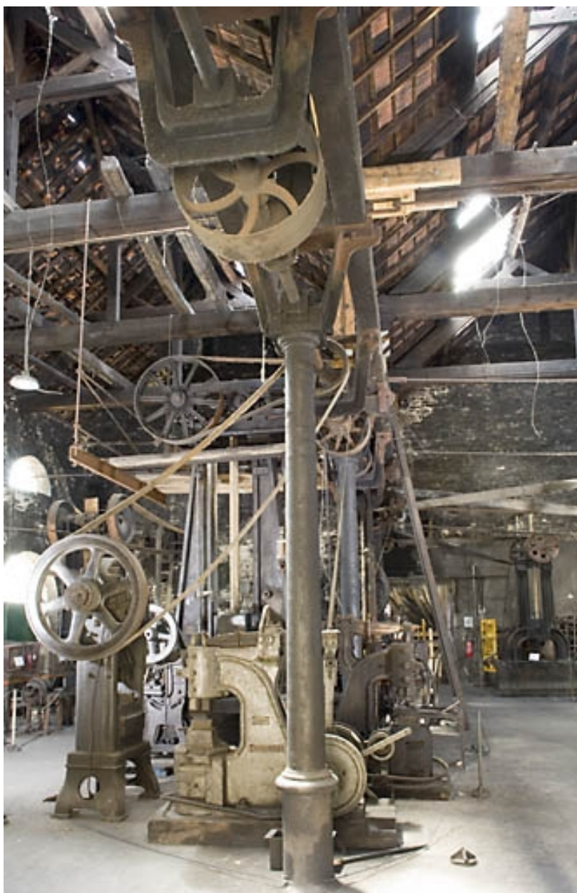
Intérieur de l'atelier est. Vue depuis l'est.
