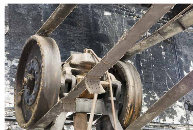
Atelier est. Marteau-pilon. Détail de la transmission supérieure par poulies et courroies. Phot. Jérôme Mongreville IVR43_20087000825NUC2A
