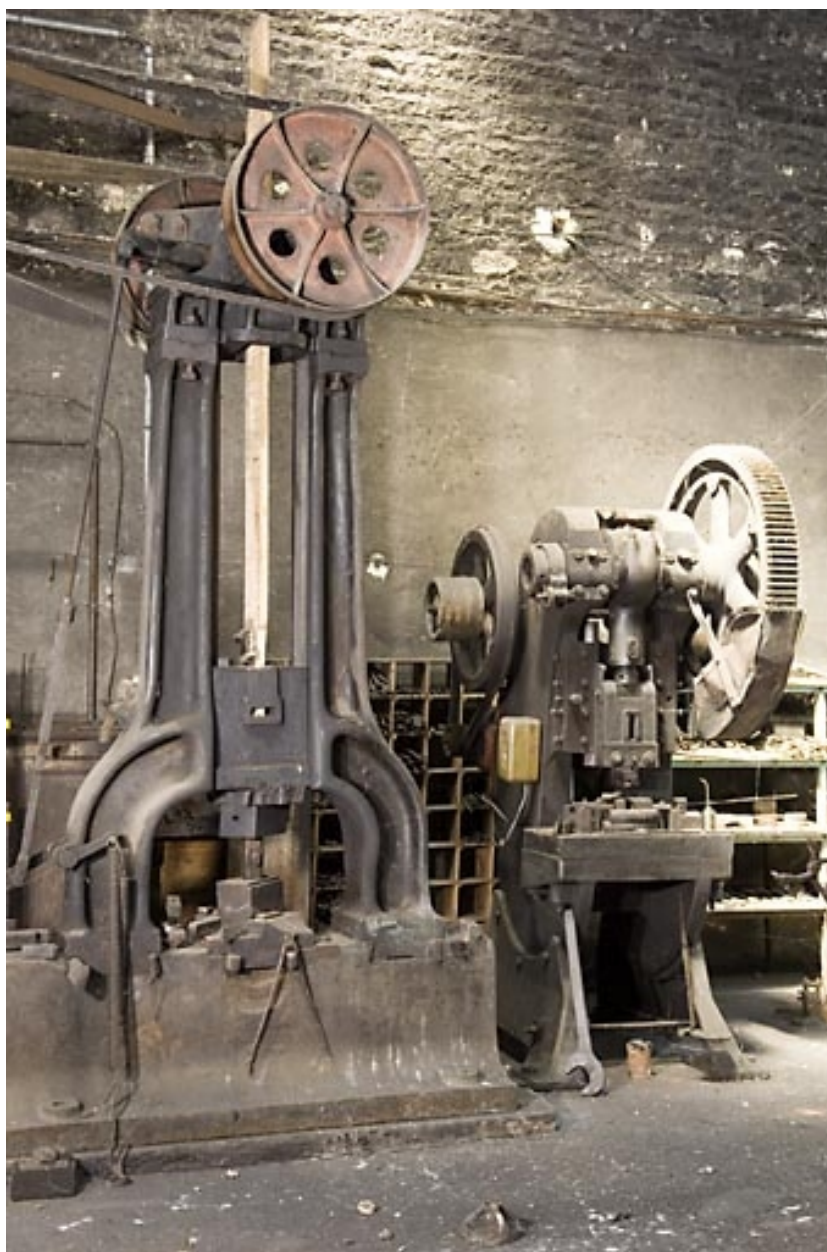
Atelier est. Marteau-pilon Delinotte (Paris) et presse "col de cygne".
