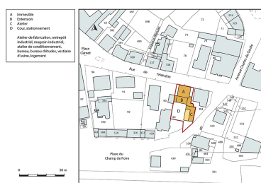
Plan-masse et de situation. Extrait du plan cadastral, 2018, section AA, 1/1 000. Dess. Bertrand Turina IVR43_20182501417NUDA
