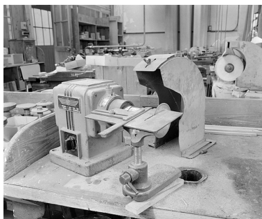
Vue d'ensemble de la scie (atelier de finissage). Phot. Jérôme Mongreville IVR43_20022500466X
