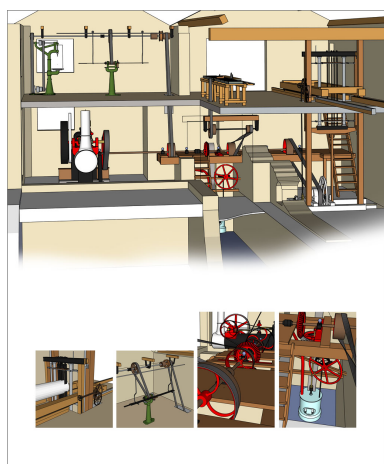
Schéma de distribution de la force motrice à la scierie Lescot (Rémondans-Vaivre). Dess. Mathias Papigny IVR43_20142500590NUDA
