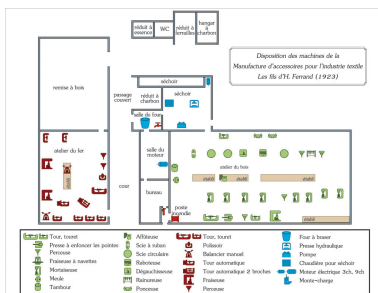
Usine de boissellerie Ferrand à Grand-Charmont. Disposition des machines (1923). Dess. Mathias Papigny IVR43_20142500592NUDA
