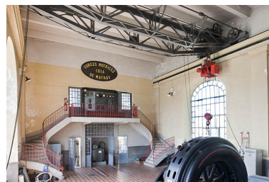
Centrale hydroélectrique de Mathay. Phot. Jérôme Mongreville IVR43_20122501786NUC4A
