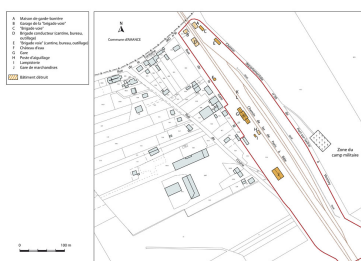
Plan-masse et de situation. Extrait du plan cadastral, 1996, section F. Dess. Mathias Papigny IVR43_20157000340NUDA
