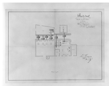
Plan de détail présenté à l'appui de la demande en maintien d'usine à Morez formée par le Sr Bruno Jacquemin.
