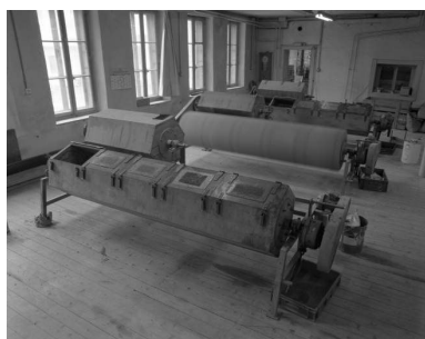
Ateliers de fabrication (1892) : tonneaux de polissage. Phot. Jérôme Mongreville IVR43_19913900856X
