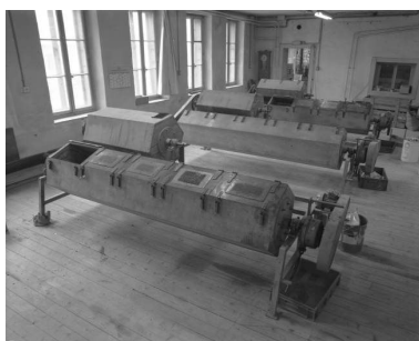
Ateliers de fabrication (1928-1929) : machines dans l'atelier à l'étage. Phot. Jérôme Mongreville IVR43_19913900852X
