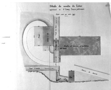
Règlement d'eau [...] Plan et dessins de détails [plan-masse du moulin]. Phot. Jérôme Mongreville, Phot. Pernot IVR43_19963900189X
