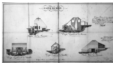
Usine de Bley [coupes et élévations du fourneau et du patouillet]. Phot. Yves Sancey, Autr. Gonzalez IVR43_19877000022X
