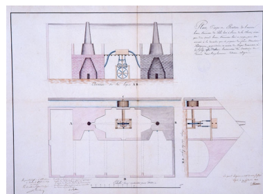
Plan, coupe et élévation de l'ancien haut fourneau de Blé [...]. Phot. Yves Sancey IVR43_19877000021XA
