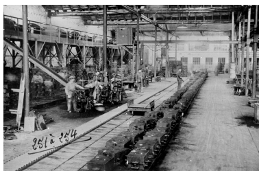
Atelier de seconde fusion. Phot. Yves Sancey IVR43_19869000022Z
