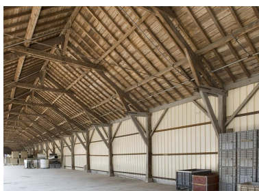
Fermes de la charpente de l'entrepôt industriel. Phot. Jérôme Mongreville IVR43_20097000733NUC2A
