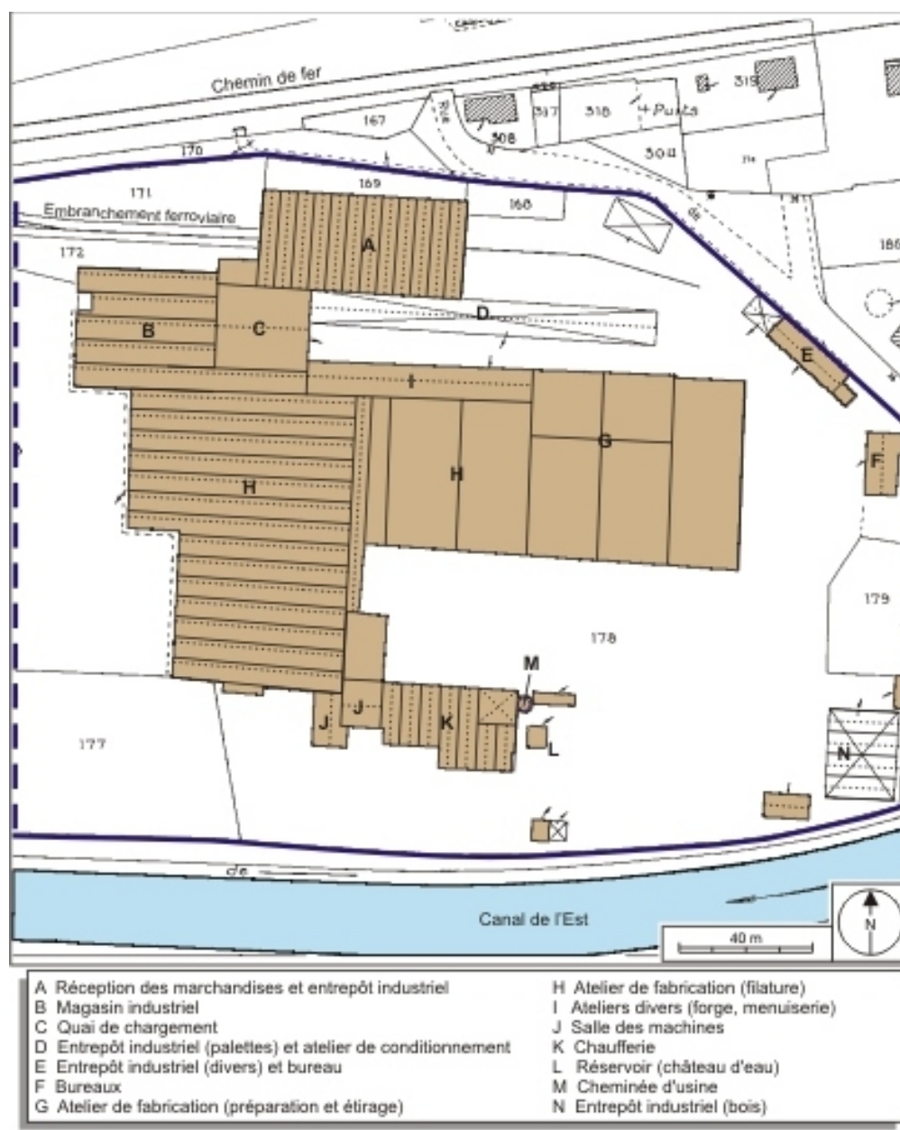
Plan-masse de l'usine. Extrait du plan cadastral numérisé, 2008, section B, 1:1250 réduit à 1:1500. Source : Direction générale des Finances Publiques - Cadastre ; mise à jour : 2008.
