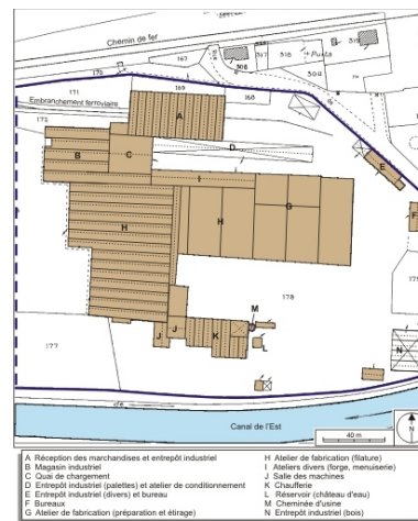
Plan-masse de l'usine. Extrait du plan cadastral numérisé, 2008, section B, 1:1250 réduit à 1:1500. Source : Direction générale des Finances Publiques - Cadastre ; mise à jour : 2008. Dess. André Céréza IVR43_20087000476NUDA
