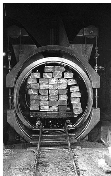
L'autoclave chargé. Phot. Laurent Poupard IVR43_19883900337Z
