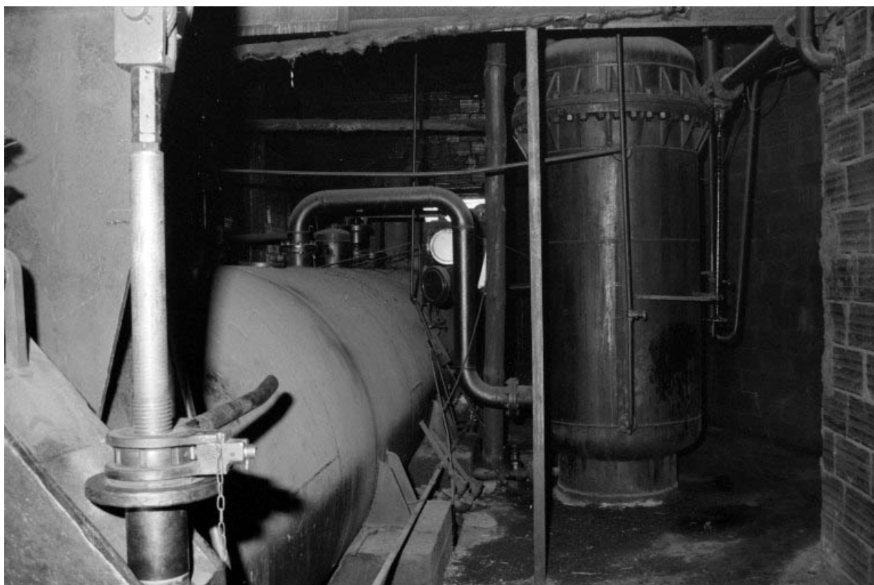
L'autoclave. Autoclave à gauche, cuve de créosote à droite.
