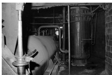
L'autoclave. Autoclave à gauche, cuve de créosote à droite. Phot. Laurent Poupard IVR43_19883900336Z
