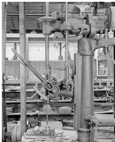
Vue rapprochée du côté droit. Phot. Yves Sancey IVR43_20022500901X
