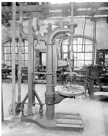
Vue d'ensemble du côté gauche. Phot. Yves Sancey IVR43_20022500898X
