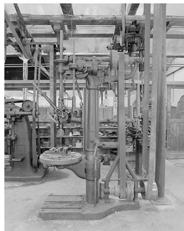
Vue d'ensemble du côté droit. Phot. Yves Sancey IVR43_20022500899X
