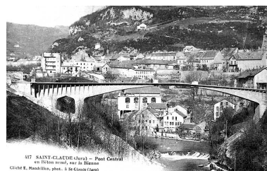
Saint-Claude (Jura) - Pont Central en Béton armé, sur la Bienne. Phot. Jérôme Mongreville, Phot. E. Mandrillon IVR43_19923900049X
