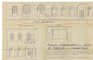
Projet d'aménagement des salles de théâtre et de gymnastique [coupe et élévations]. S.d. [1948]. Phot. Pierre-Marie Barbe- Richaud, Autr. Armand Inconnu IVR26_20245800371NUC4A
