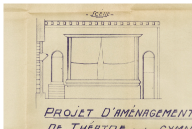
Projet d'aménagement des salles de théâtre et de gymnastique [coupe et élévations : détail de la scène]. S.d. [1948]. Phot. Pierre-Marie Barbe- Richaud, Autr. Armand Inconnu
