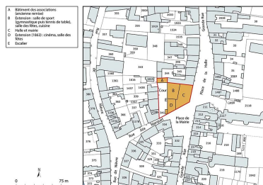
Plan-masse et de situation. Source : Direction générale des Finances Publiques - Cadastre ; mise à jour 2024, section C, 1/1 000. Dess. Aline Thomas IVR26_20245800764NUDA
