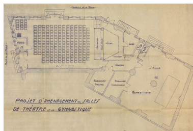
Projet d'aménagement des salles de théâtre et de gymnastique [plan]. S.d. [1948]. Phot. Pierre-Marie Barbe- Richaud, Autr. Armand Inconnu IVR26_20245800370NUC4A
