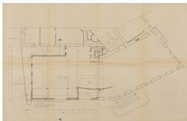
Ville de Prémery. Projet d'agrandissement de la salle des fêtes. 1. Plan du 1 er étage. Février 1970. Phot. Pierre-Marie Barbe- Richaud, Autr. Armand Inconnu, Autr. Daniel Chenut IVR26_20245800368NUC4A
