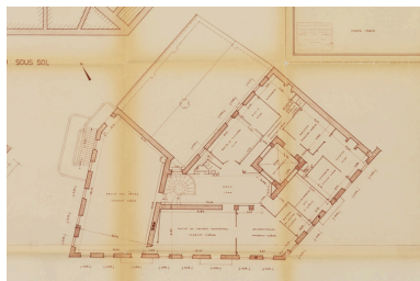
Ville de Prémery. Mairie. Plans état actuel. Plan du premier étage. Mars 1963. Phot. Pierre-Marie Barbe- Richaud, Autr. Armand Inconnu IVR26_20245800366NUC4A
