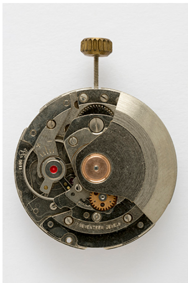
Mouvement France Ebauches FE 5611 : face côté ponts. Phot. Sonia Dourlot IVR43_20162500750NUC4A
