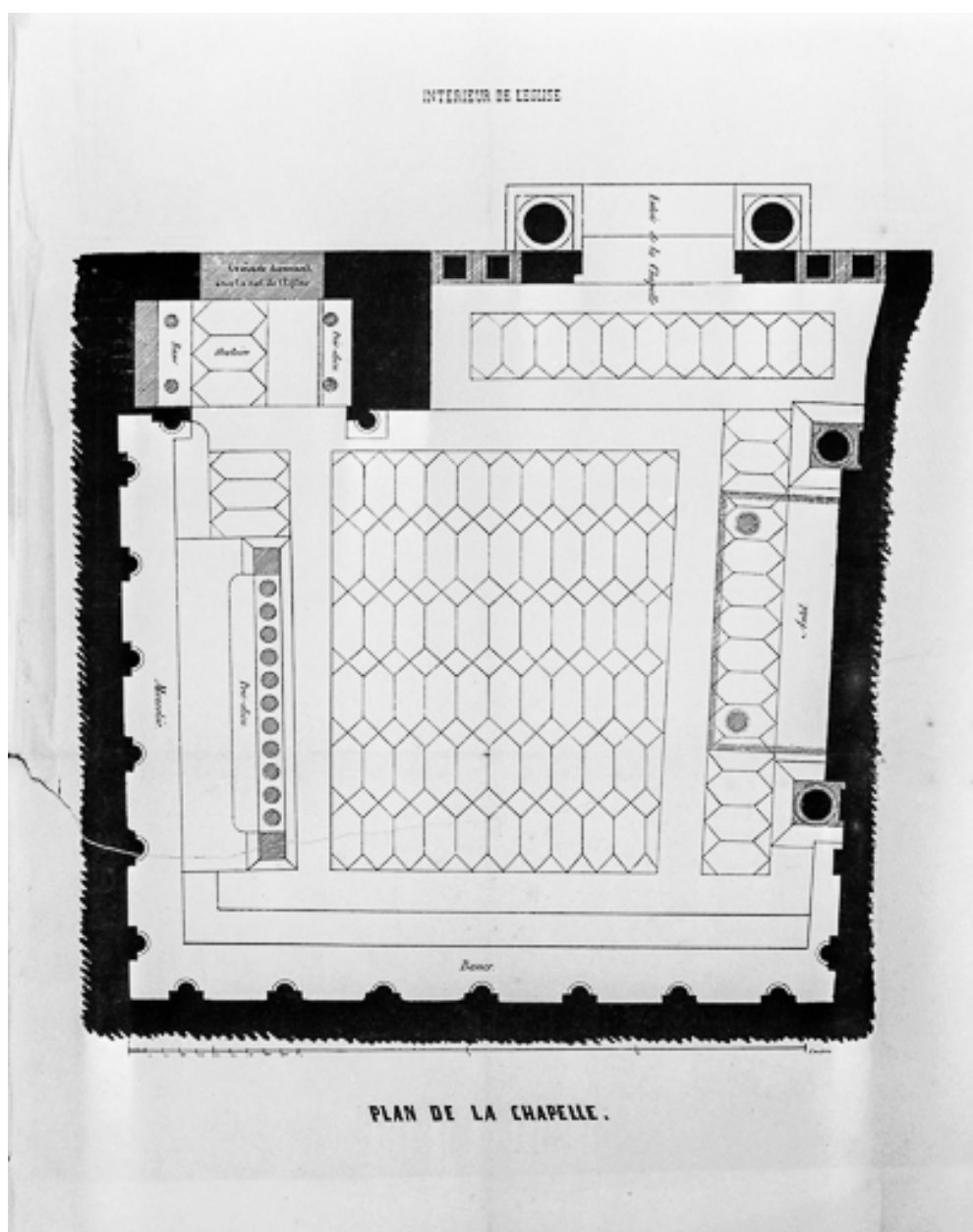
Plan de la chapelle de la Résie.
