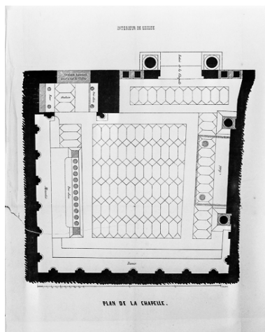
Plan de la chapelle de la Résie. Phot. Yves Sancey IVR43_19847000006V
