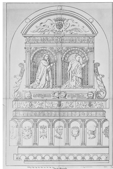
Face du mausolée : projet de restauration. Phot. Yves Sancey IVR43_19847000011V
