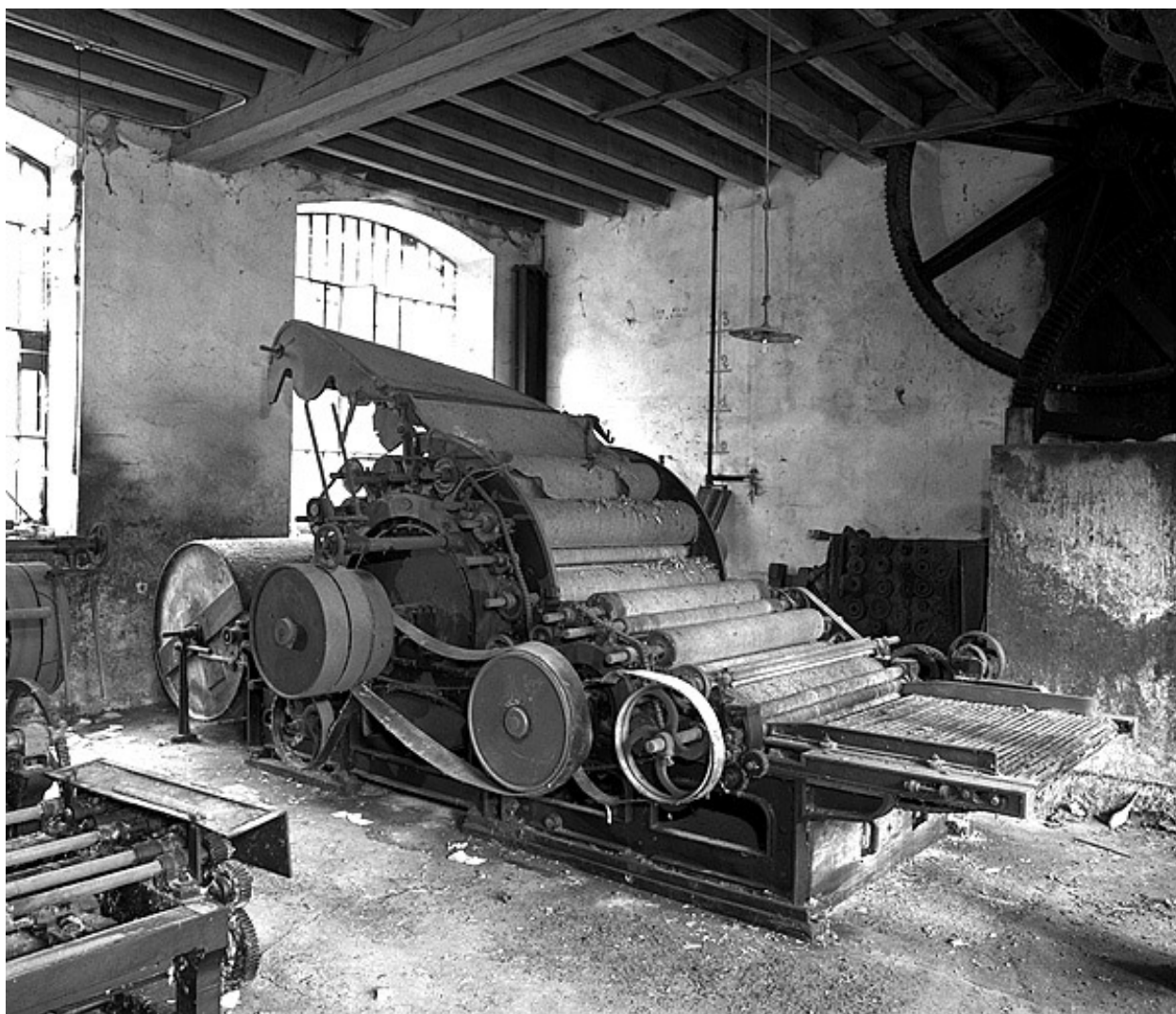
Vue d'ensemble.
