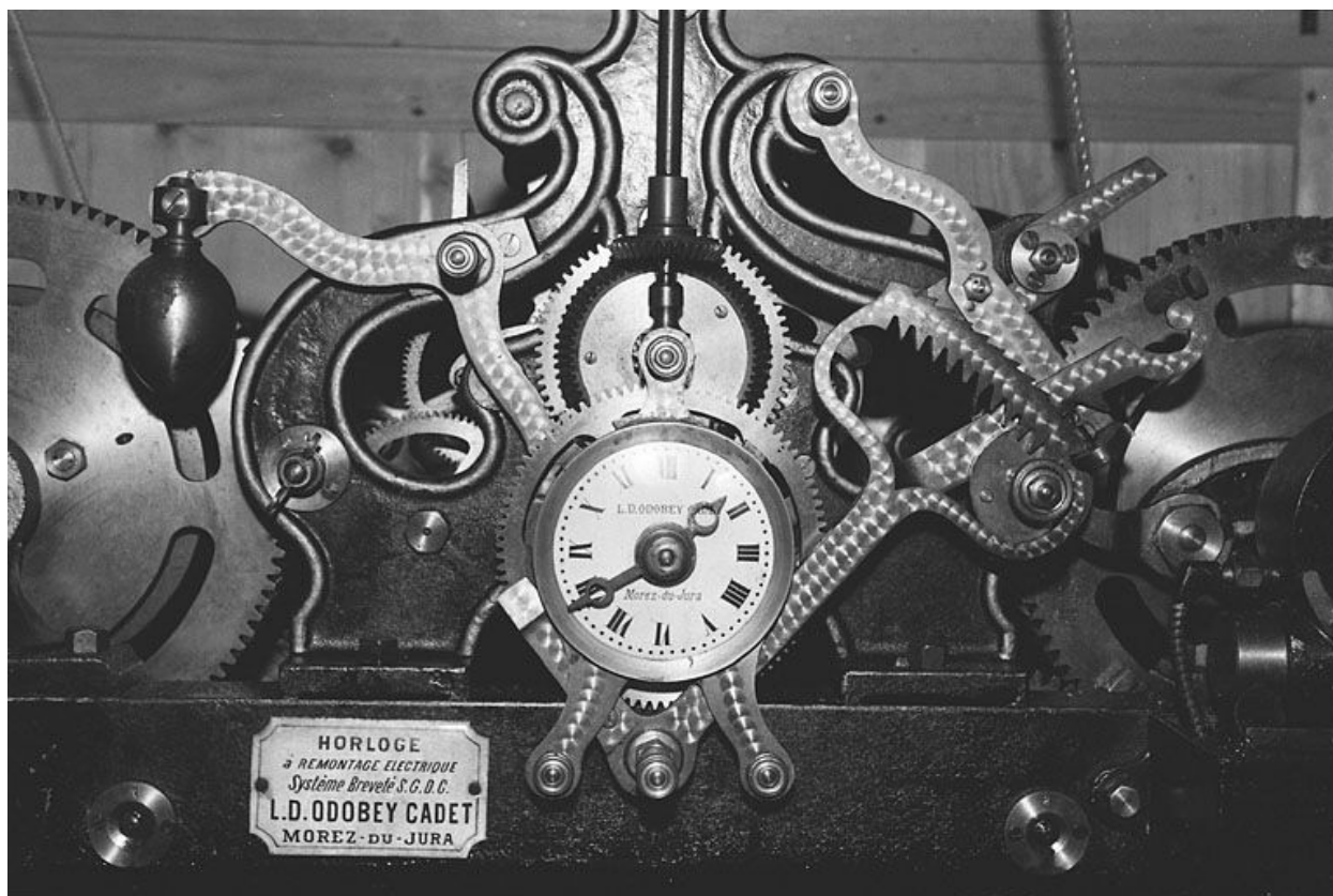
Partie centrale du mouvement.
