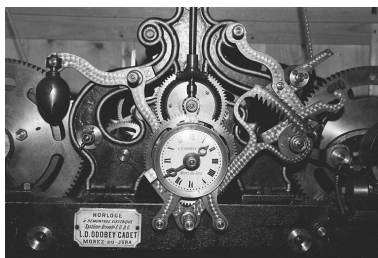
Partie centrale du mouvement. Phot. Jérôme Mongreville IVR43_20003900761Z
