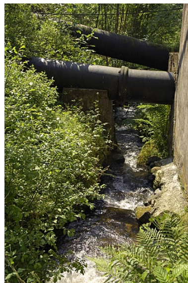
Arrivée des conduites forcées. Phot. Jérôme Mongreville IVR43_20057000344NUCA
