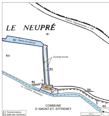
Plan-masse et de situation. Extrait du plan cadastral numérisé, 2005, section C, 1:2500 agrandi à 1:1000. Dess. André Céréza IVR43_20067000015NUDA
