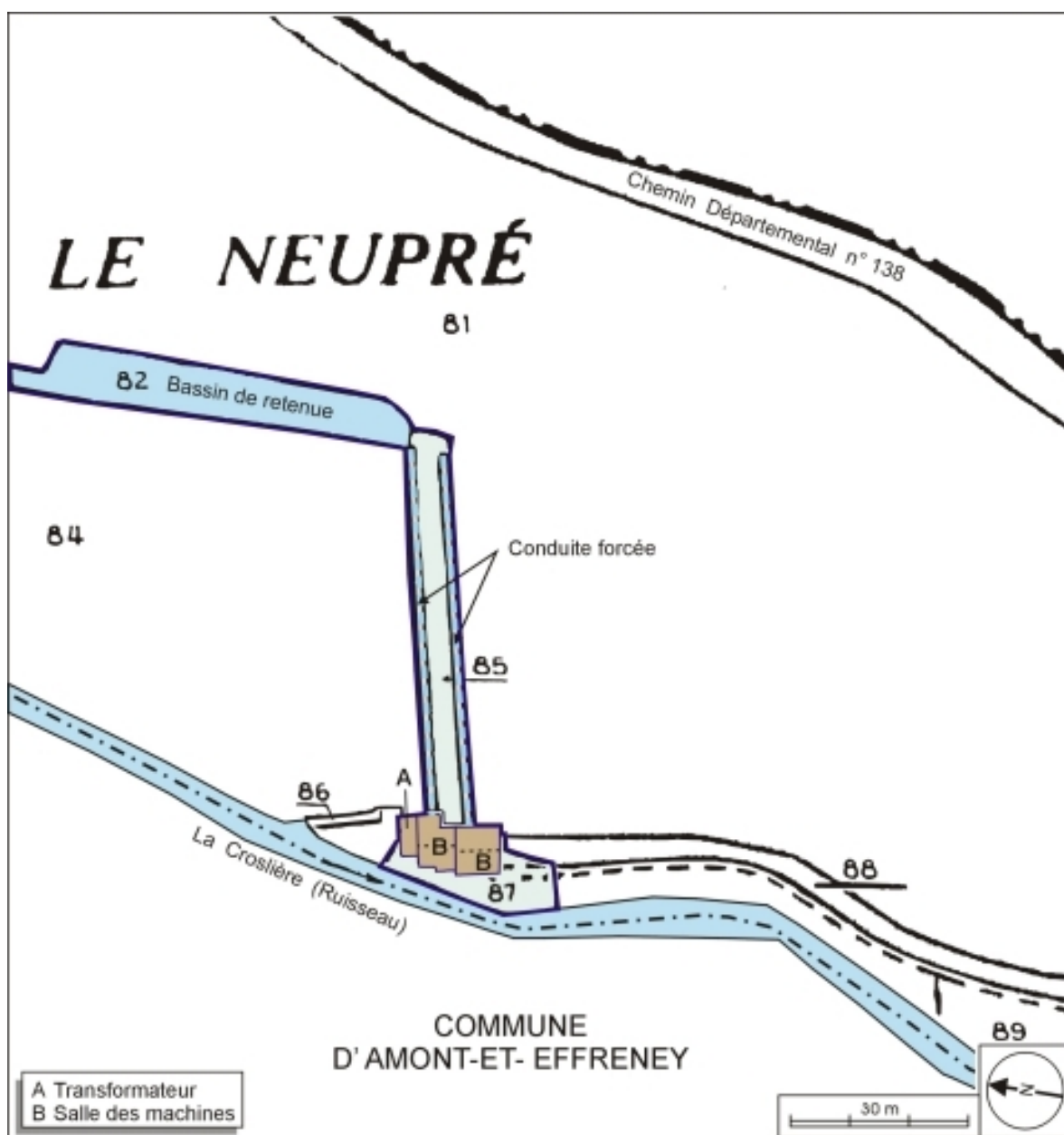
Plan-masse et de situation. Extrait du plan cadastral numérisé, 2005, section C, 1:2500 agrandi à 1:1000.
