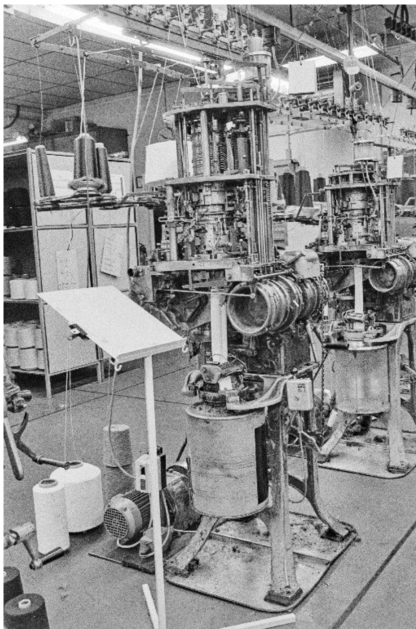
Machine à tricoter des chaussettes dite " Komet ", de type LT : vue d'ensemble.
