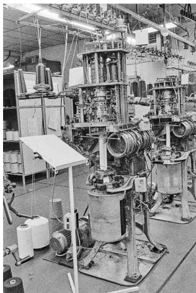
Machine à tricoter des chaussettes dite " Komet ", de type LT : vue d'ensemble. Phot. Frédéric Pillet IVR26_19997100255Z
