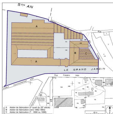
Plan-masse et de situation. Extrait du plan cadastral, 1984, section AL, 1:1000 réduit à 1:1500. Dess. André Céréza IVR43_20039000018NUDA
