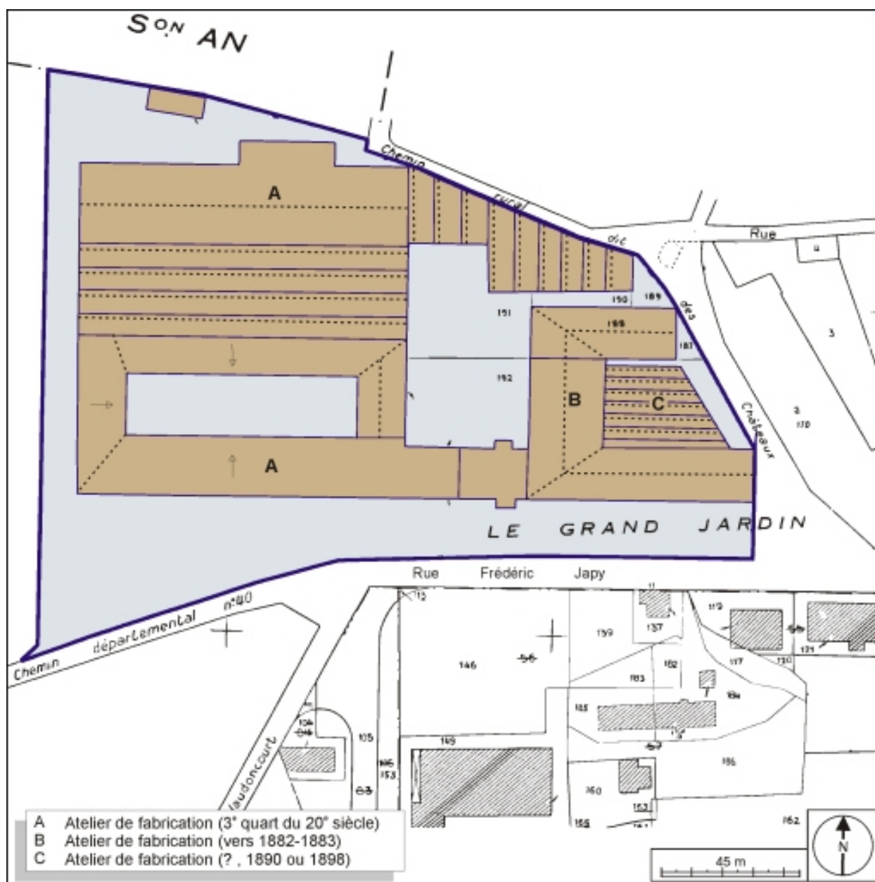
Plan-masse et de situation. Extrait du plan cadastral, 1984, section AL, 1:1000 réduit à 1: 1500.
