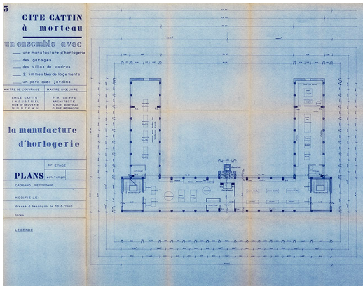
Cité Cattin à Morteau [...] 3. La manufacture d'horlogerie. Plans 1er étage. Cadrans, nettoyage, 10 juin 1960.
