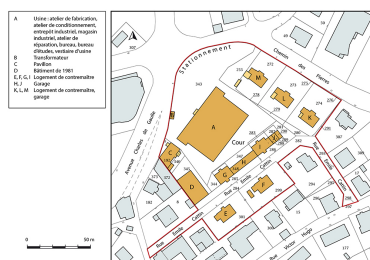
Plan-masse et de situation. Extrait du plan cadastral, 2018, section AF, 1/1 000. Dess. Bertrand Turina IVR43_20182501427NUDA
