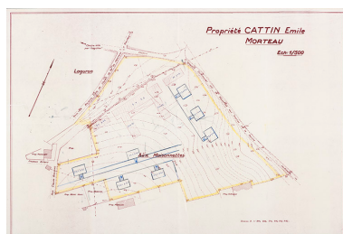
Propriété Cattin Emile [plan-masse et de situation], Morteau, 1960 ? Phot. Sonia Dourlot IVR43_20192500851NUC4A
