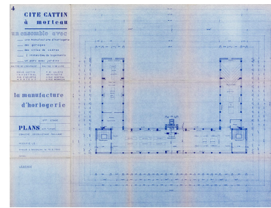
Cité Cattin à Morteau [...] 4. La manufacture d'horlogerie. Plans 2ème étage. Ebauche, décolletage, taillage, 10 juin 1960. Phot. Sonia Dourlot IVR43_20192500845NUC4A
