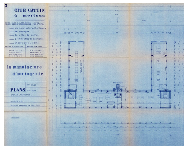
Cité Cattin à Morteau [...] 3. La manufacture d'horlogerie. Plans 1er étage. Cadrans, nettoyage, 10 juin 1960. Phot. Sonia Dourlot IVR43_20192500846NUC4A
