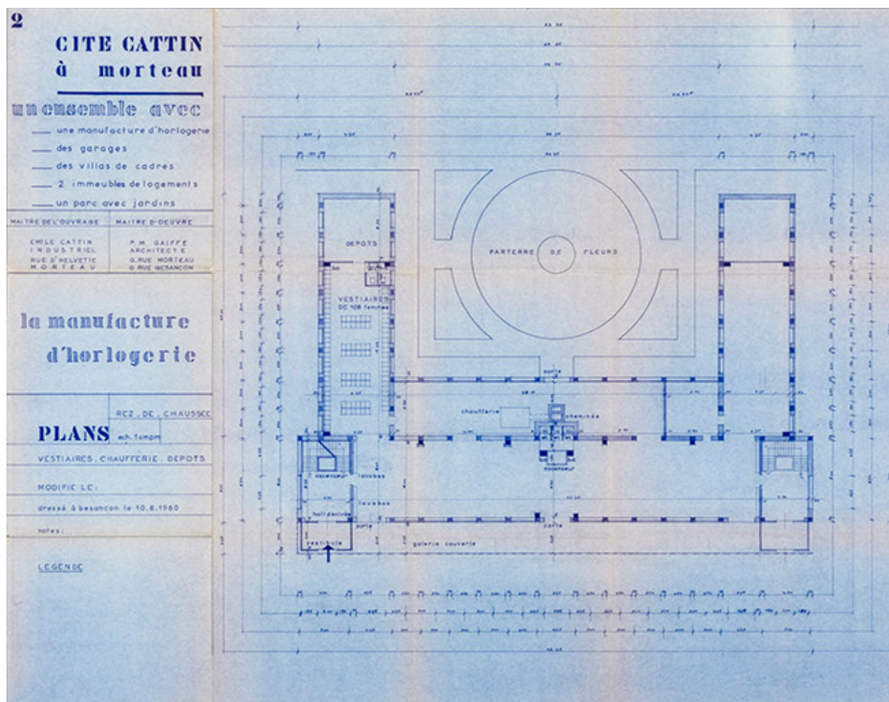
Cité Cattin à Morteau [...] 2. La manufacture d'horlogerie. Plans rez-de-chaussée. Vestiaires, chaufferie, dépôts, 10 juin 1960.
