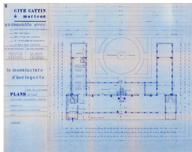
Cité Cattin à Morteau [...] 2. La manufacture d'horlogerie. Plans rez-de-chaussée. Vestiaires, chaufferie, dépôts, 10 juin 1960. Phot. Sonia Dourlot IVR43_20192500847NUC4A
