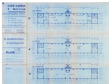
Cité Cattin à Morteau [...] 5. La manufacture d'horlogerie. Plans 3e étage [bureaux], 4e étage [finition], 5e étage [expédition], 10 juin 1960. Phot. Sonia Dourlot IVR43_20192500844NUC4A
