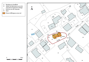
Plan-masse et de situation, section AB. Dess. Mathias Papigny IVR43_20142501926NUDA
