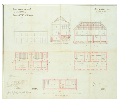
Commune de Fallérans. Construction d'une maison d'école [plans, coupes et élévation], 1849. Phot. Jérôme Mongreville IVR43_20152500592NUC4A
