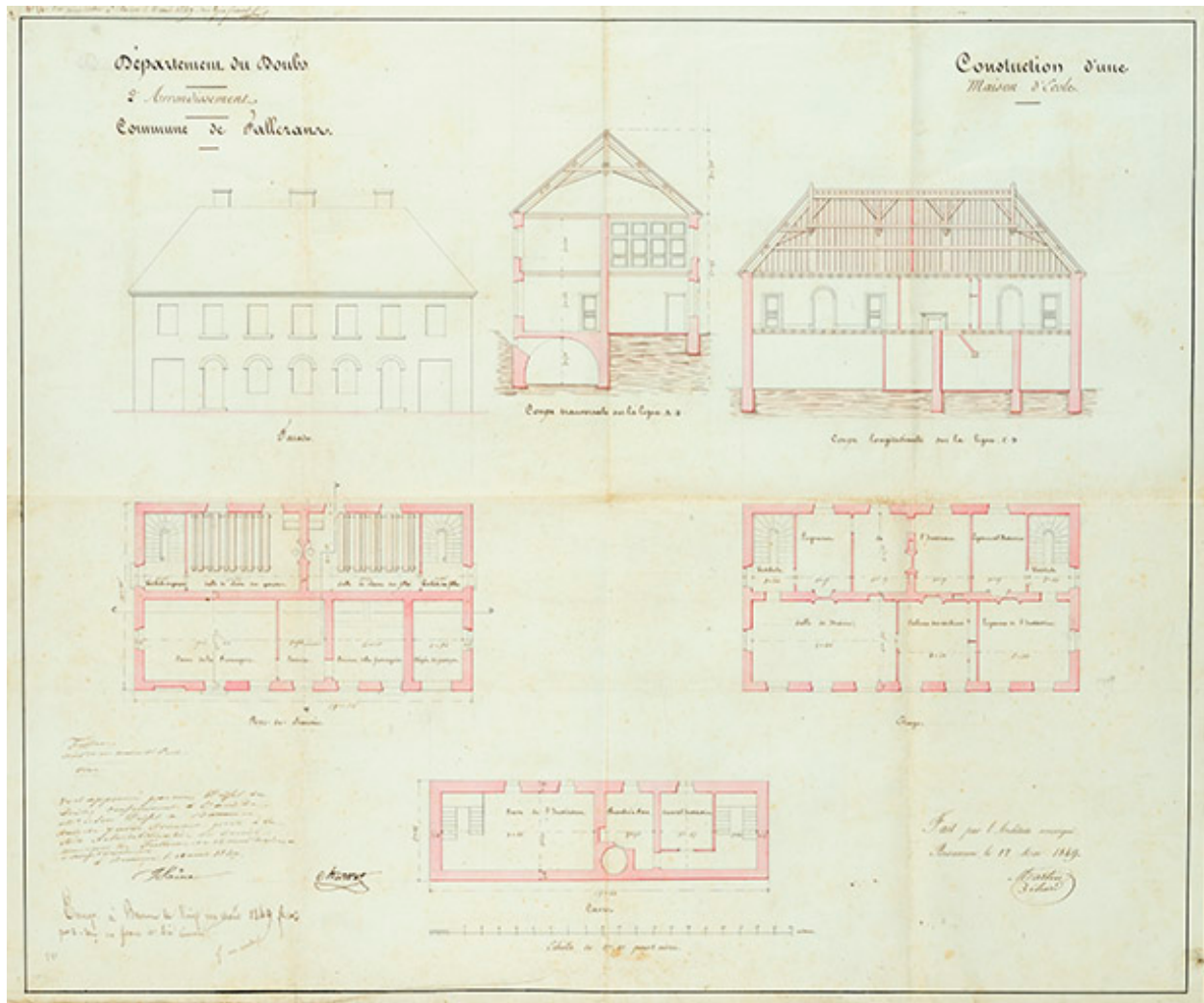
Commune de Fallerans. Construction d'une maison d'école [plans, coupes et élévation], 1849.
