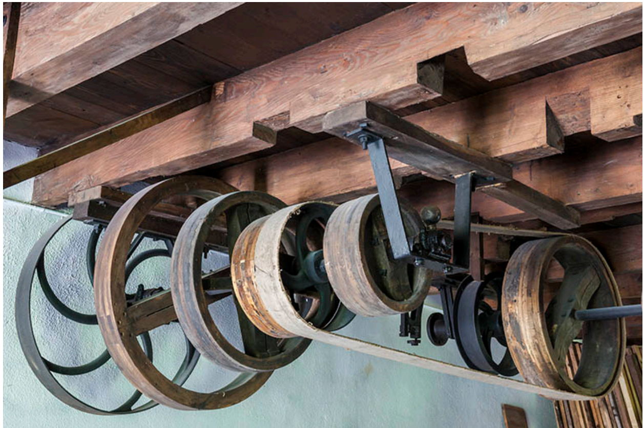
Détail de la transmission par poulies.
