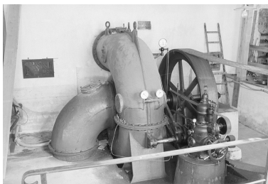
Turbine Schneider Jacquet et Cie. Phot. Laurent Poupard IVR43_19913901154Z
