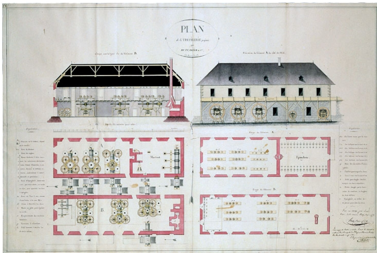
Plan de la Tréfilerie projetée par Rutly Ogier, et Cie de Morez - Jura.
