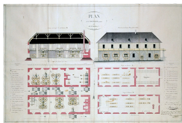
Plan de la Tréfilerie projetée par Ruty Ogier, et Cie de Morez - Jura. Phot. Jérôme Mongreville, Autr. Louis (industriel) NEPASUTILISEROgier IVR43_19943900378VA
