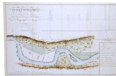
Plan et nivellemens du Cours de la Bienne entre le Moulin de la Daraise et la Tréfilerie des Srs Ruty Ogier et Comp. Phot. Jérôme Mongreville IVR43_19943900382VA
