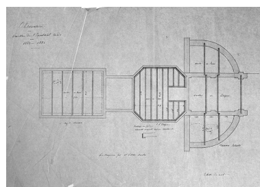
Pavillon de l'équatorial coudé. Poutrage en fer et petites voûtes [plan], 1883-1884. Phot. Yves Sancey IVR43_20042500211X
