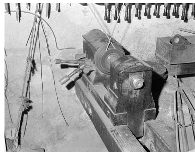
Tour à marchepied : clavier et clés de sélection. Phot. Jérôme Mongreville IVR43_19963901048X
