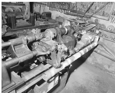
Tour automatique, permettant de travailler la galalithe, datant de 1920 environ. Phot. Jérôme Mongreville IVR43_19963901056X
