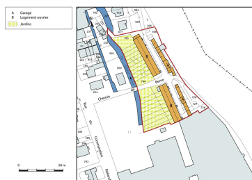
Plan-masse et de situation. Dess. Mathias Papigny IVR43_20132502636NUDA
