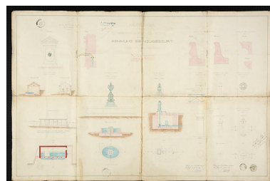
Construction de fontaines. [plan et élévation] 1867 Phot. Sonia Dourlot IVR43_20167000110NUC4A
