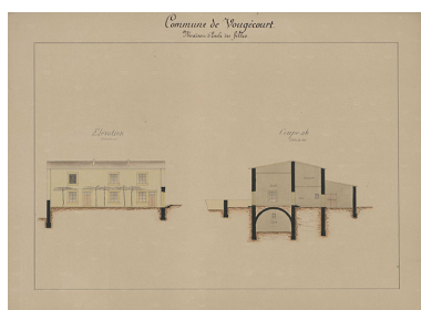
Plans des écoles (1864 -1888) : élévation et coupe de l'école de filles. Phot. Philippe Mairot IVR43_20167000157NUC4A
