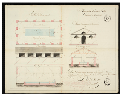
Projet de lavoir couvert. [plan, coupes et élévations] 1825 Phot. Sonia Dourlot IVR43_20167000116NUC4A
