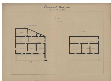
Plans des écoles (1864 -1888) : plan de l'école de filles. Phot. Philippe Mairot IVR43_20167000156NUC4A
