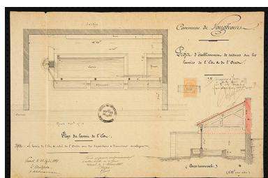
Projet d'établissement de toitures sur les lavoirs. [plans et coupes] 1887 Phot. Sonia Dourlot IVR43_20167000108NUC4A
