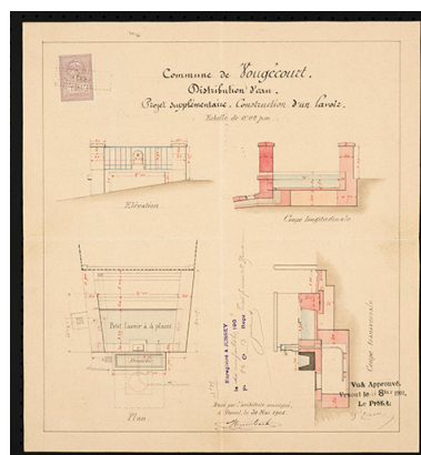
Distribution en eau, construction d'un lavoir. [plan] 1901 Phot. Sonia Dourlot IVR43_20167000107NUC4A
