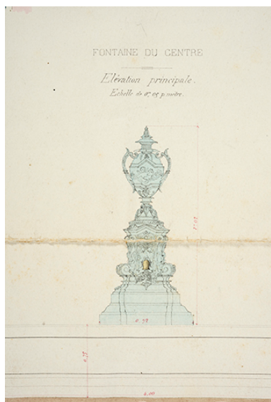
Fontaine du centre. Elévation principale. [Détail du plan] 1867 Phot. Sonia Dourlot IVR43_20167000111NUC4A
