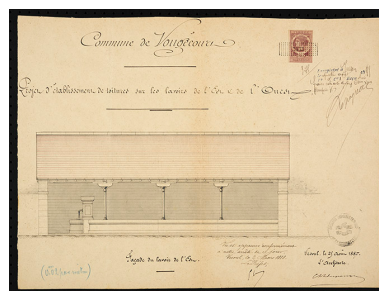
Projet d'établissement de toitures sur les lavoirs de l'est et de l'ouest. [Élévation] 1887 Phot. Sonia Dourlot IVR43_20167000109NUC4A
