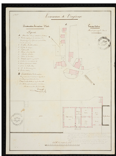
Construction d'une maison d'école et mairie. [plan] 1852 Phot. Sonia Dourlot IVR43_20167000114NUC4A
