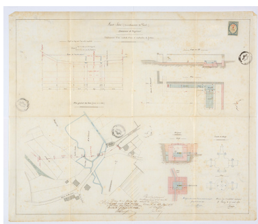
Etablissement d'une conduite d'eau et construction de fontaines, plan général des lieux. [plan, coupes, élévations] 1878 Phot. Sonia Dourlot IVR43_20167000123NUC4A
