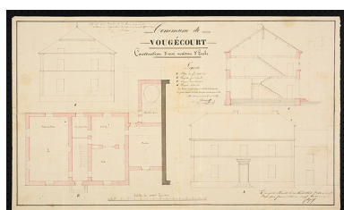
Construction d'une maison d'école et mairie. [plan, coupes et élévations] 1852 Phot. Sonia Dourlot IVR43_20167000115NUC4A
